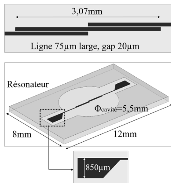
Figure 10. Dimensions de la conception du résonateur micro-ruban
