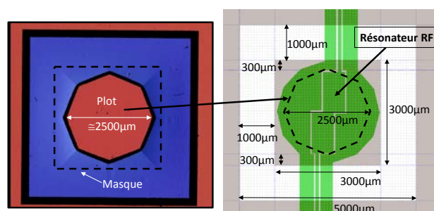
Figure 3. Photo de la membrane (gauche) et dessin des masques (droite)
