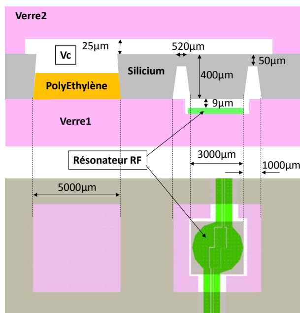
Figure 2. Vue en coupe (dessus) et dessin des masques (dessous) du capteur
