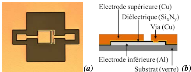
Figure 5. Capacité de test de 11 pF. (a) Photographie et (b) vue en coupe longitudinale.
