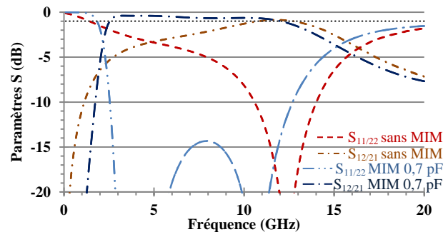
Figure 3. Paramètres S du transformateur 4 tours adapté 50Ω-50Ω.
