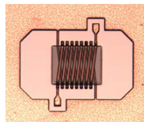
Figure 1. Photographie du transformateur à 2 enroulements de 4 spires (vue de dessus).
