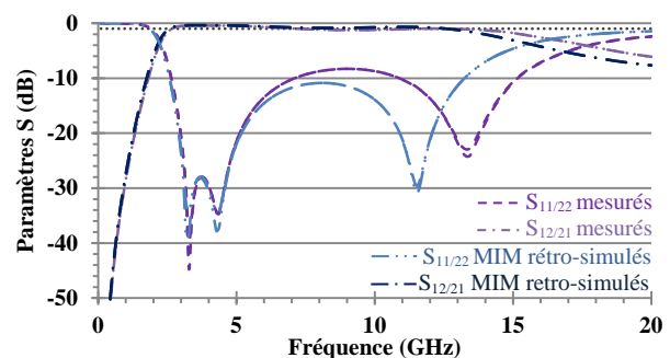
Figure 7. Paramètres S rétro-simulés et mesurés pour le transformateur 4 tours adapté 50 \Omega -50 \Omega .
