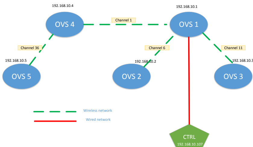
FIGURE 3.10: Contrôle In-band.
