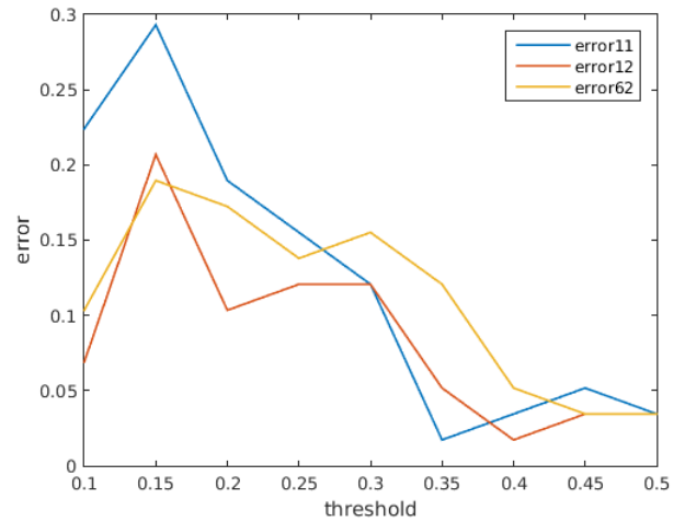
FIGURE 8 – Taux d'erreur de classification
