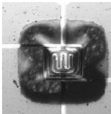
Figure 7 : Effet de la géométrie du heater sur le comportement mécanique de la plateforme de la génération précédente.
