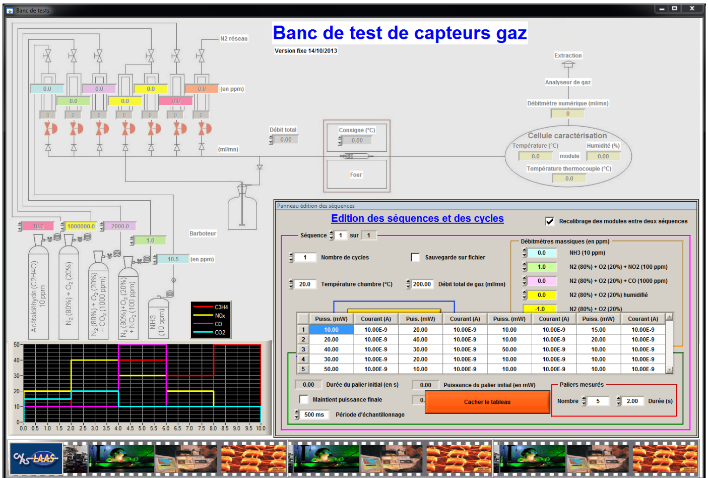
Fig. 4 : Interface utilisateur développée avec LabWindows/CVI
