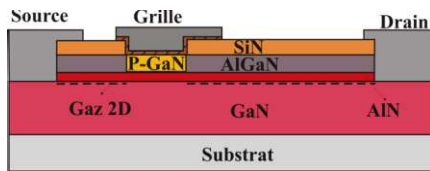
Fig. 1. Structure d'un HEMT en GaN avec une grille à barrière P-GaN
