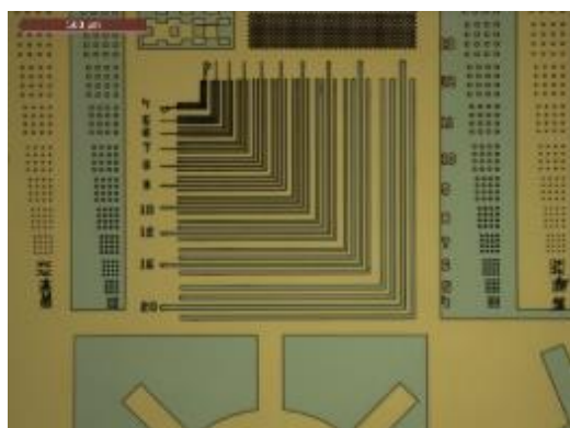
Figure 6 résine négative AZ125NXT épaisseur 30μm pour la gravure du silicium
