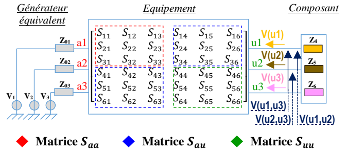
Fig. 8. Injection de mode commun sur l'équipement
