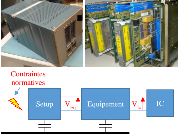
Fig. 1. Exemple d'équipement aéronautique (en haut) ; Propagation d'une perturbation à un composant
