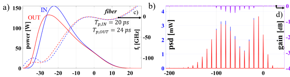
Fig 3. Résultat numérique illustrant le profil en régime stationnaire d'une impulsion optique (a) et de sa dsp associée (b) avant (IN) et après (OUT) la traversée du tronçon fibré de longueur L 1 (β 2Σ,1 = -0.89 ps 2 ). L'évolution des impulsions optiques a été étudiée de la même manière à la traversée de chacun des composants de la boucle optique (SOA, MZM, fibre dispersive, filtre passe-bande).
