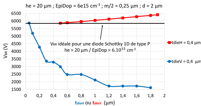
Fig. 5 : Variation de la tenue en tension en fonction de t dieH ou t dieV pour t dieV = 0,4 μm (courbe en Blue) et t dieH = 0,4 μm (courbe en Rouge) respectivement à 300 K.
