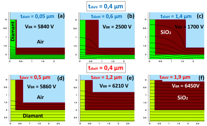
Fig. 6 : Représentation des lignes équipotentielles au moment du claquage en fonction de t dieH ou t dieV pour t dieV = 0,4 μm (Blue) et t dieH = 0,4 μm (Rouge) respectivement à 300 K
