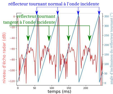
Figure 2. Niveau d'écho radar mesuré à la distance radar-réflecteur (courbe rouge) et angle d'inclinaison (courbe bleue) en fonction du temps.
