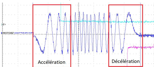
Courant dans une des bobines d'un moteur pas à pas, onde de courant sinusoïdale
