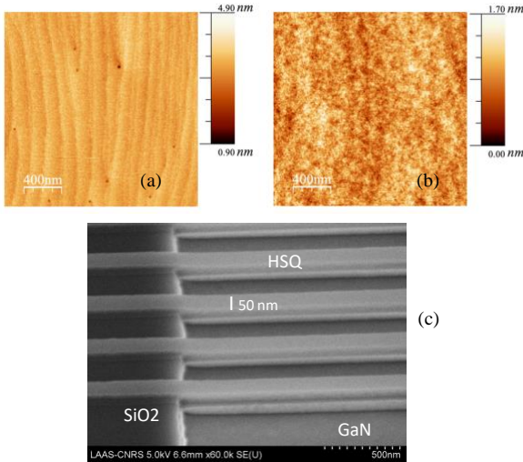
Fig. 7. Mesures AFM montrant la rugosité de surface des couches GaN loin (a) et près (b) des bords de caisson ; Observation MEB de nano-fils de HSQ/GaN de 50 nm de large (c).
