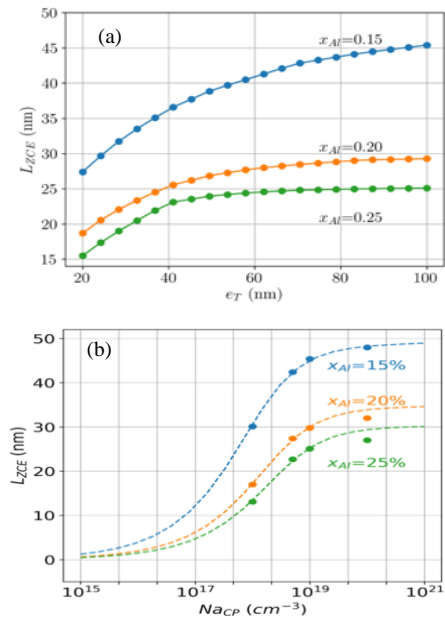
Fig. 4. Variations de L_{ZCE} en fonction de e_T pour Na_{CP} fixé à 1 \times 10^{19} cm^{-3} (a) et en fonction de Na_{CP} pour e_T fixé à 100 nm (b) pour différents d'aluminium x_{Al} dans l'AlGaIn de 15%, 20% et 25%.
