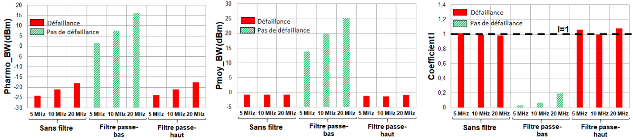
Fig.5. Seuil de susceptibilité conduite à une perturbation large bande de la référence de tension
