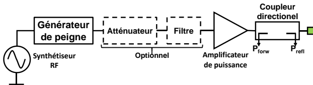
Fig.3. Chaîne d'injection large bande
