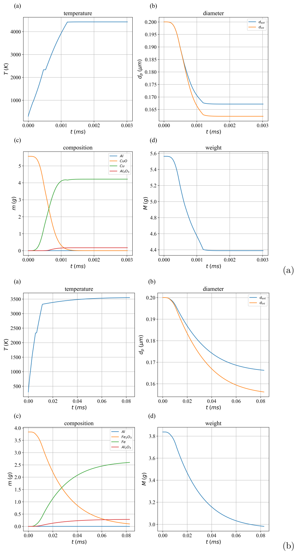
FIGURE VI.8 – Cas nanométrique (2.) Résultats obtenus pour la phase particulaire d'oxyde métallique pour les nanothermites (a) Al/CuO et (b) Al/Fe_2O_3
