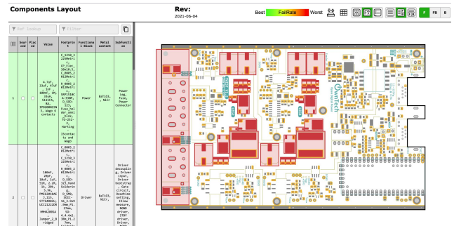
Figure 9 - Capture d'écran montrant les composants du groupement fonctionnel « Bloc Puissance » soulignés en rouge
