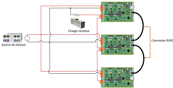
Figure 6 - Schéma de trois cartes OwnTech connectées en parallèle pour augmenter le courant fourni à la charge
