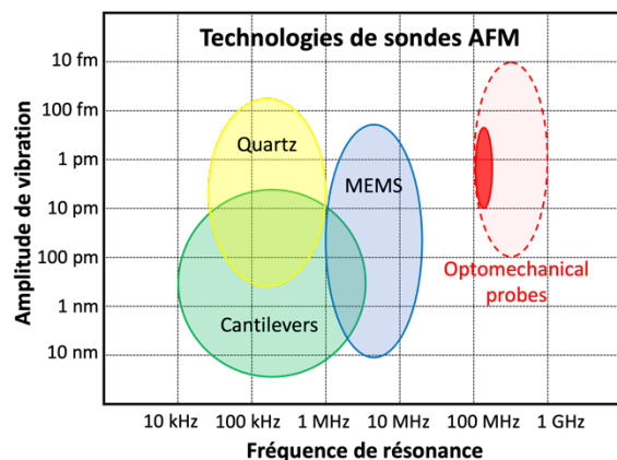
Figure 1 : à gauche, les technologies existantes de sondes AFM pour le mode dynamique. Les ellipses représentent les gammes d'amplitude de vibration et de fréquence de résonance atteintes par chaque technologie. A droite, une image en microscopie électronique à balayage d'une sonde AFM optomécanique fonctionnant à la fréquence de 130 MHz. Figure adaptée de [2].
