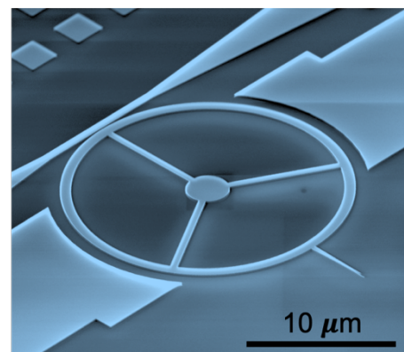
Figure 1 : à gauche, les technologies existantes de sondes AFM pour le mode dynamique. Les ellipses représentent les gammes d'amplitude de vibration et de fréquence de résonance atteintes par chaque technologie. A droite, une image en microscopie électronique à balayage d'une sonde AFM optomécanique fonctionnant à la fréquence de 130 MHz. Figure adaptée de [2].
