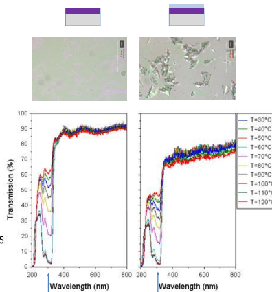
Bande spectrale de suivi de la transition SCO
