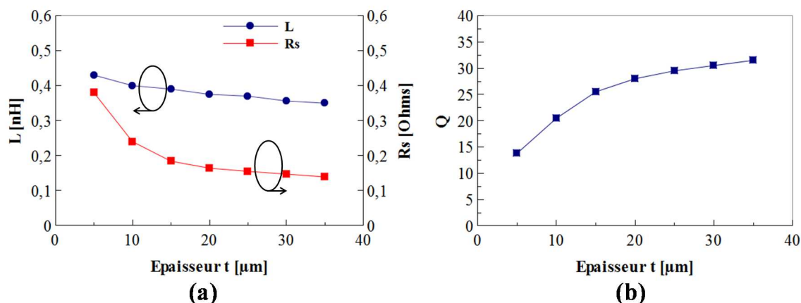
Figure II.8 : variations (a) de l'inductance L , de la résistance série R_s et (b) du facteur de qualité Q à 2 GHz en fonction de l'épaisseur de conducteur t (inductance de 1 tour, W=30 \mu\text{m} ).
