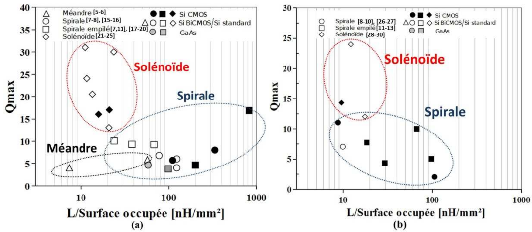
Figure I.11 : état de l'art pour les inductances (a) et les transformateurs (b) RF intégrés représenté sous la forme du facteur de qualité maximal Q_{\text{max}} en fonction de la valeur d'inductance L par unité de surface occupée.
