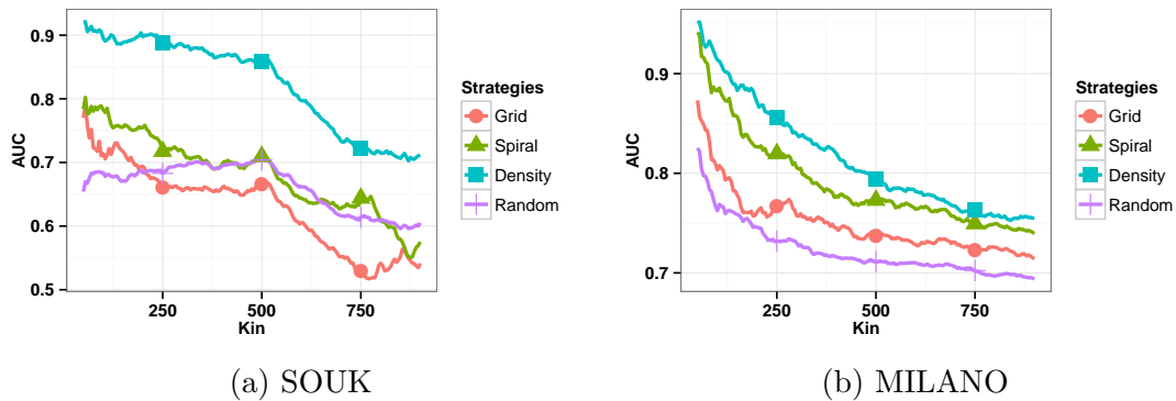
FIGURE 3.5 – L’impact de K_{in} dans les données SOUK (a) et MILANO (b), avec un déploiement de 15 capteurs de portée 1m .
