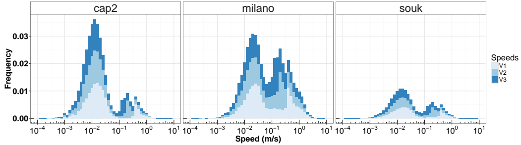
FIGURE 2.8 – Histogramme avec les densités de fréquences des vitesses dans les données réelles avec \Delta t \in [1, 2, 3] .
