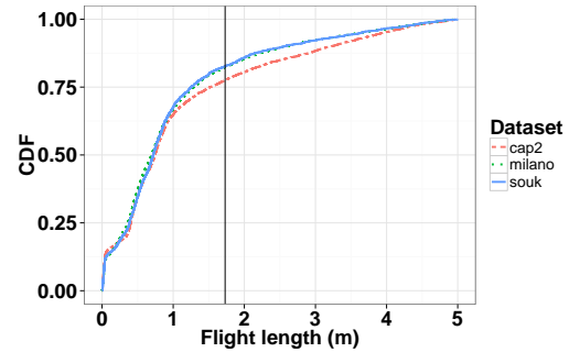
FIGURE 2.10 – Fonction de répartition de la distance franchissable dans le cas des données réelles.
