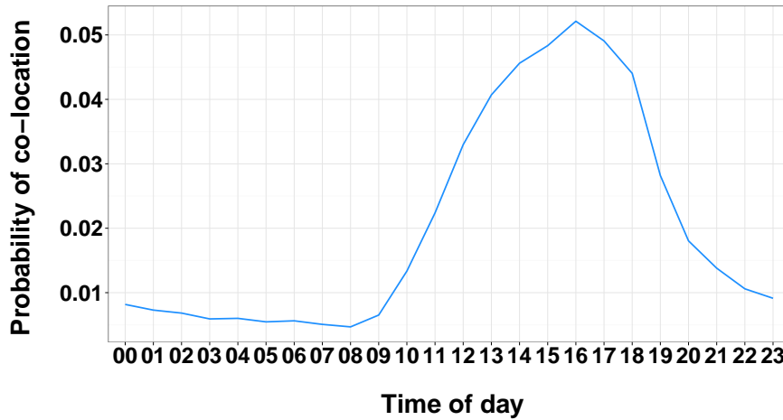
FIGURE 4.2 – Profil probabiliste de co-localisation moyenné sur l’ensemble des couples d’utilisateurs.
