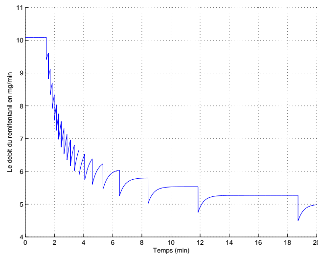
FIGURE 7.4 – Le débit de rémifentanyl injecté en boucle fermée avec le Contrôleur 1 ( \Delta = 1 )
