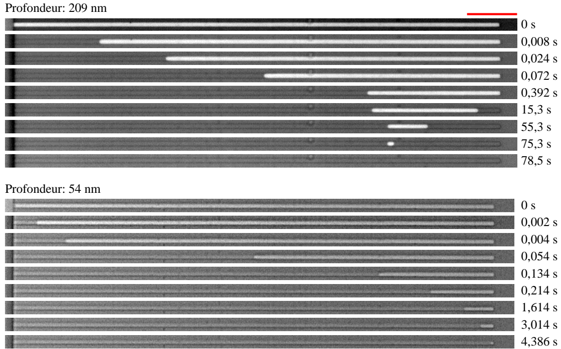
FIGURE 3.18 – Comparaison de la cinétique d’imbibition de nanocanaux en impasse de 209 nm et 54 nm de profondeur. L’échelle de longueur représente 100 \mu\text{m} .
