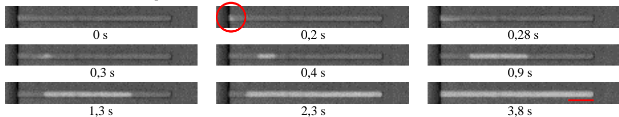
FIGURE 3.26 – Apparition d'une bulle lors de l'évaporation d'éthanol dans un nanocanal de 300\ \mu\text{m} de longueur. a) Canal de 209 nm de profondeur. b) Canal de 54 nm de profondeur. Le cercle rouge souligne l'apparition de la bulle. L'échelle de longueur représente 50\ \mu\text{m} dans le sens du canal. L'image est dilatée dans la direction transversale afin de mieux voir le phénomène (le canal fait 4\ \mu\text{m} de large).
