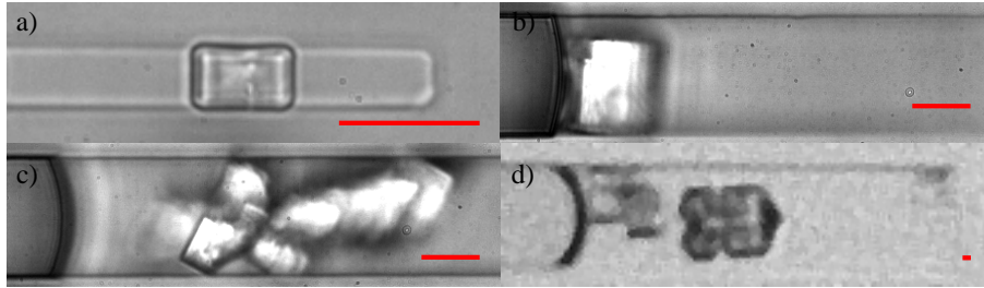
FIGURE 4.7 – Formes des cristaux de NaCl lors la croissance dans une solution sursaturée. a) Une forme quasi-cubique est observée dans les canaux de 5 \times 5 \mu\text{m}^2 . b) et c), la forme du cristal dans un canal de 20 \times 20 \mu\text{m}^2 dépend du degré de confinement géométrique. Si le cristal est confiné entre le ménisque et la paroi du pore, le cristal est quasi-cubique. Lorsqu'il apparaît au milieu du canal, il croît avec une forme d'étoile. Dans les canaux de 50 \times 100 \mu\text{m}^2 , plusieurs cristaux croissent en même temps. L'échelle de longueur représente 10 \mu\text{m} .
