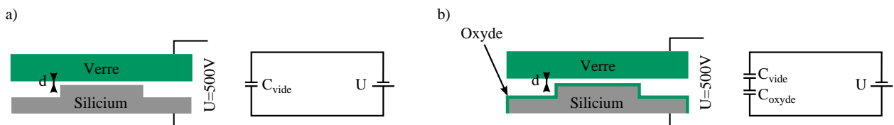
FIGURE 2.9 – Schéma représentant l'analogie entre l'assemblage des deux wafers et un condensateur plan. Cette analogie permet de calculer la pression électrostatique qui déforme les wafers lors de la soudure anodique.
