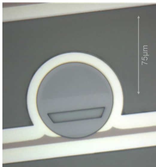
Figure IV. 13 : Image au microscope optique d'un micro-disque de 75 \mu\text{m} de diamètre (Calvez, et al., 2015)
