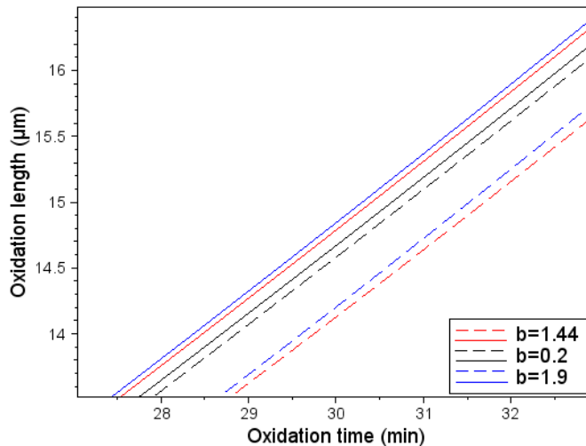
Figure III.19 : Influence du paramètre b pour une longueur d'oxydation autour de 15 µm
