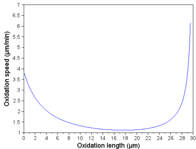
Figure III. 3 : Vitesse d'oxydation d'un mesa circulaire de 60 \mu\text{m} de diamètre en fonction de la position - Paramètres ( k=467 , h=24.6 , D=84 , C^*/N=6 ) correspondent à une oxydation d'AlAs à 400°C (Koley, et al., 1997)
