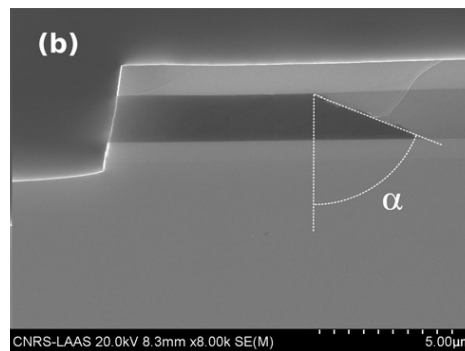
Figure II.9 : Observation MEB par la tranche d'une couche d'AlAs oxydé à 420°C pendant 30 minutes (Chouchane, et al., 2014)
