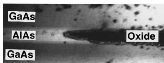
Figure II.10: Observation au microscope à effet tunnel du front d'oxydation d'une couche de 10 nm de AlAs oxydée à 450°C pendant 80 minutes (R. L. Naone, 1997)
