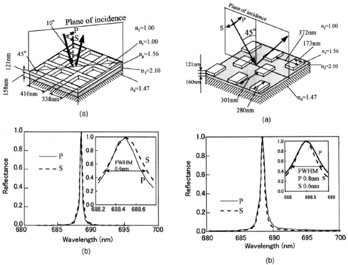
Figure 1.18 – Filtres à réseau 2D indépendants de la polarisation : à gauche est le réseau avec une maille rectangulaire : (a) structure du filtre et (b) sa réponse spectrale, à droite est le réseau avec une maille losange : (a) structure du filtre et (b) sa réponse spectrale [25].
