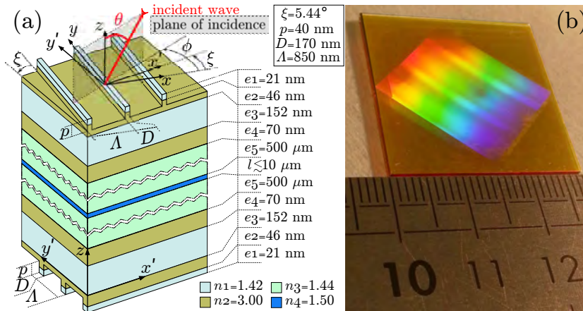
Figure 3.1 – Filtre à réseaux 1D croisés : (a) schéma de la structure, où \Lambda est le pas de réseau et D est la largeur de crête (le reste des paramètres est présenté dans la section 2.2 du deuxième chapitre) (b) photo du filtre réalisé [4].
