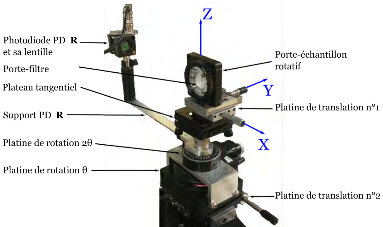
Figure 4.2 – Montage porte-échantillon.
