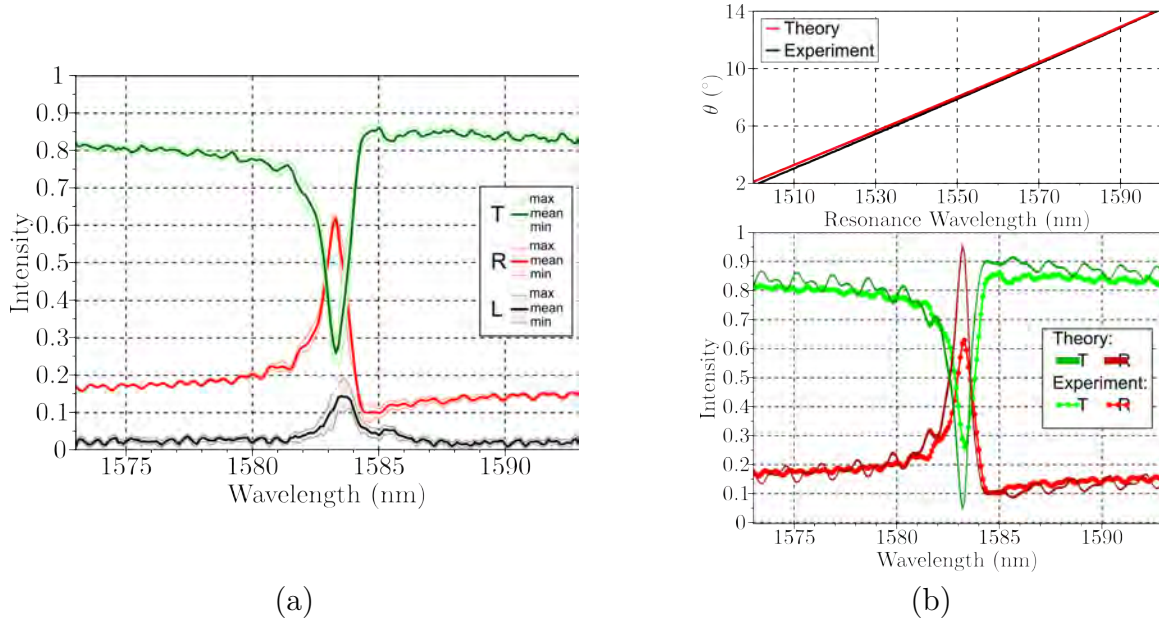
Figure 3.2 – Réponses spectrales du filtre à réseaux 1D croisés : (a) indépendance à la polarisation : en réflexion (R, rouge, courbe au milieu), en transmission (T, vert, courbe en haut) et pertes (L, noir, courbe en bas), (b, haut) courbe d'accordabilité en fonction de l'angle d'incidence : expérience (noir) et théorie (rouge), (b, bas) comparaison théorie/expérience pour les coefficients de réflexion (R, rouge, courbes en bas) et transmission (T, vert, courbes en haut) : expérience (courbe pointillée) et théorie (courbe lisse) [4].
