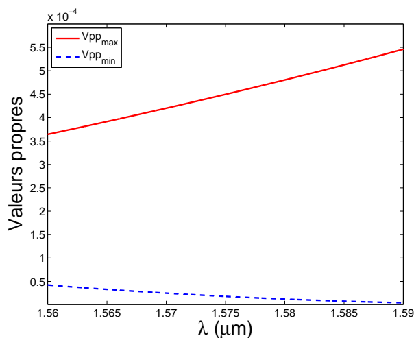
Figure 2.9 – Borne de la réflectivité inférieure ( V_{pp_{\min}} ) et supérieure ( V_{pp_{\max}} ) en fonction de la longueur d'onde lorsque la polarisation prend tous les états possibles pour l'empilement 6 couches avec profondeur de réseau h = 60 nm à l'incidence oblique de 7^\circ pour la structure avec une couche réseau homogène anisotrope.
