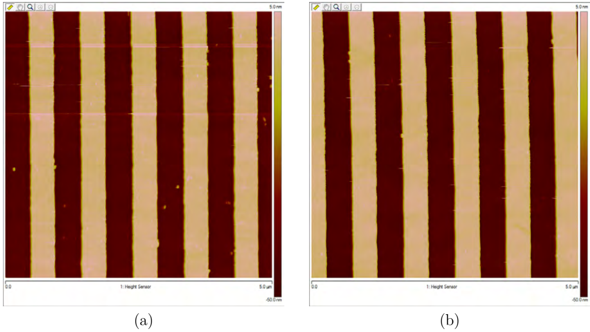
Figure 3.26 – Image AFM des échantillons après gravure de la silice est délaquage : (a) deuxième demi-filtre et (b) troisième demi-filtre.
