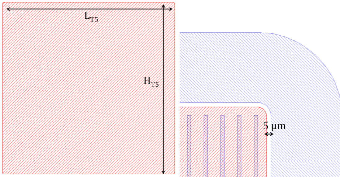
Figure A.6 : Masque négatif d'ouverture des contacts
