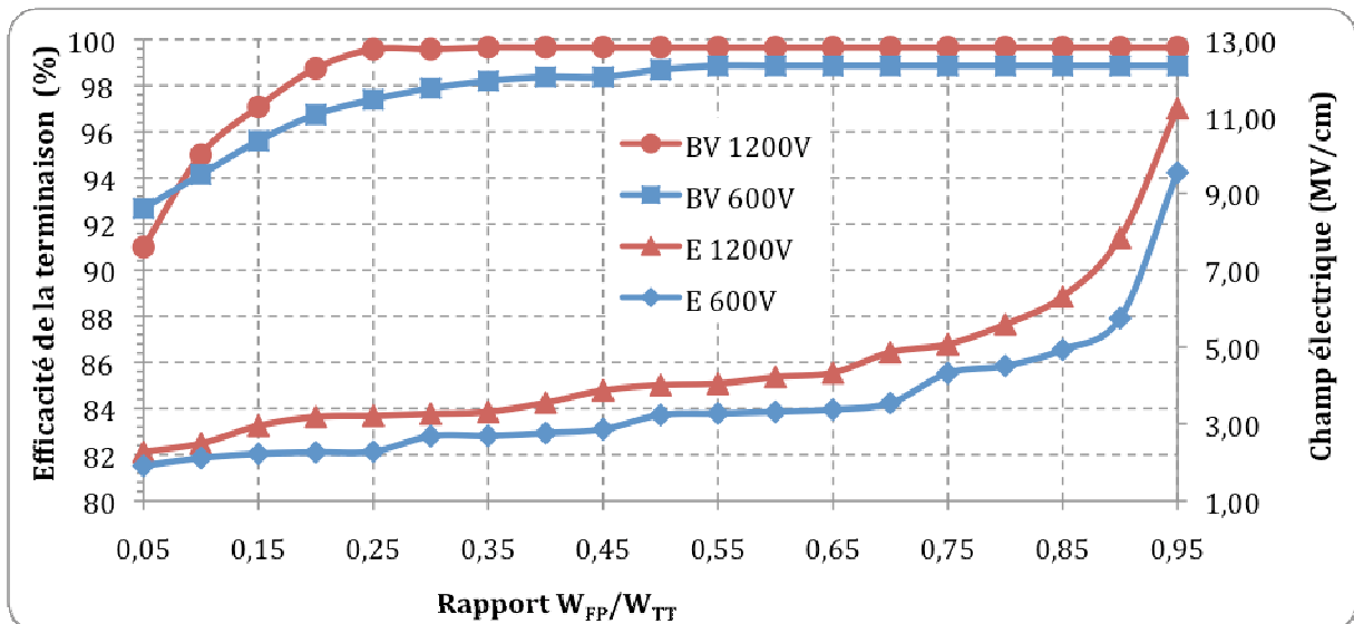
Figure II.17 : Variations de l'efficacité de la terminaison et du champ électrique au point A en fonction du rapport W_{FP}/W_{TT} pour des tenues en tension de 600V et 1200V
