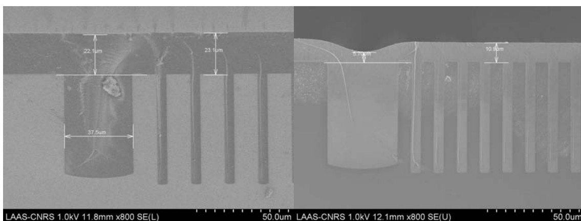
Figure III.20 : Image MEB d'un dépôt de BCB à 1500 \text{ tr/min} (à gauche) et 2000 \text{ tr/min} (à droite) suivi d'une étape de nano-impression pour des terminaisons de 40 \mu\text{m} de large
