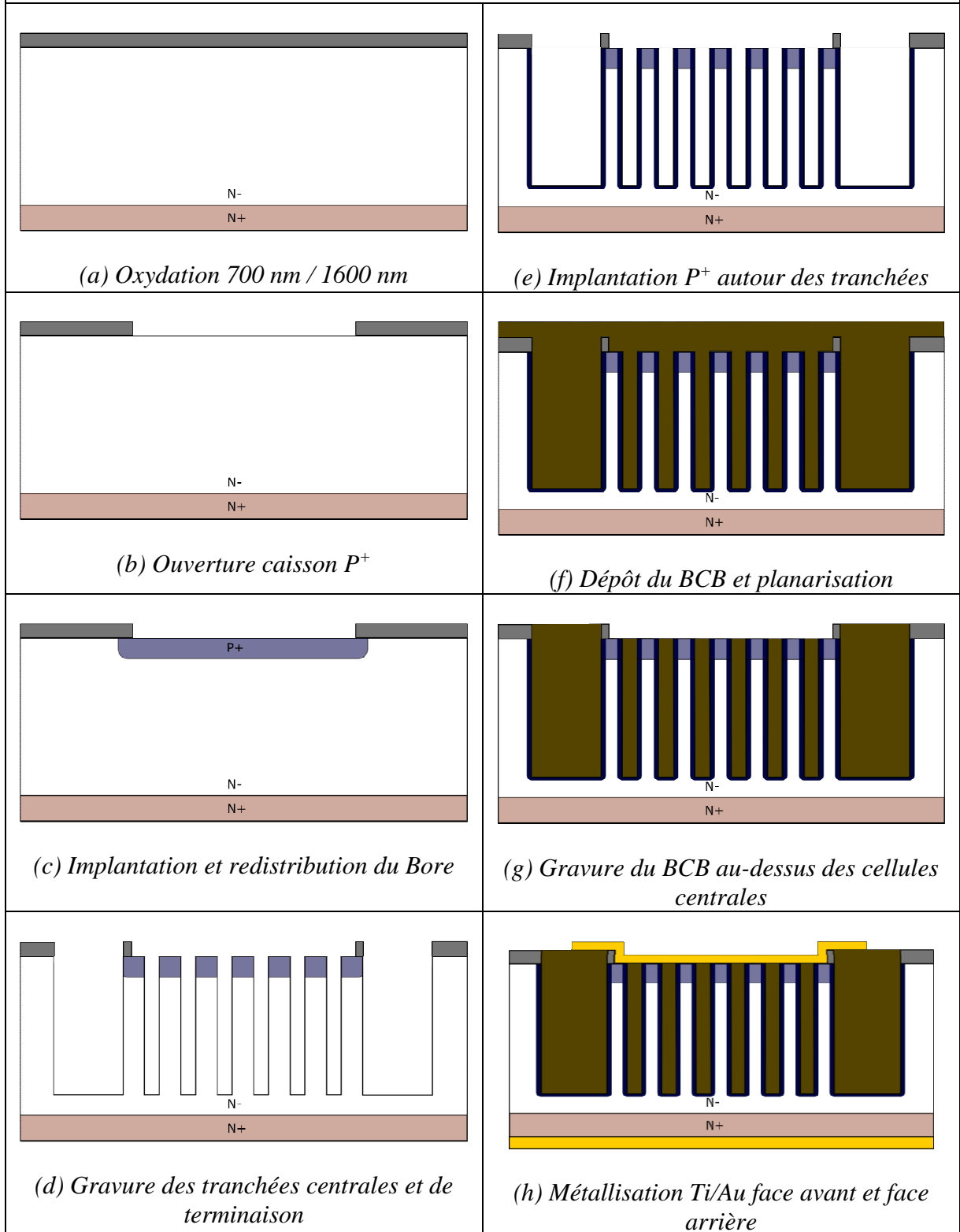
Figure IV.1 : Principales étapes de fabrication de la diode à superjonction et à tranchées profondes
