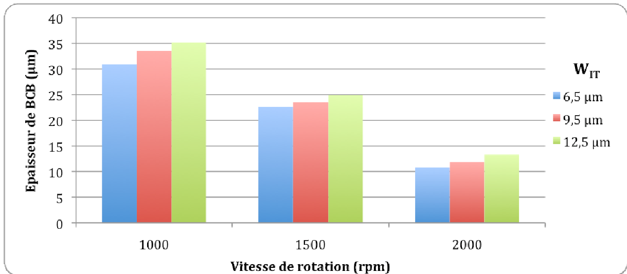
Figure III.19 : Epaisseur du BCB mesurée après nano-impression au-dessus des cellules centrales pour différentes valeurs de rotation lors du dépôt et différents espacements inter-tranchées
