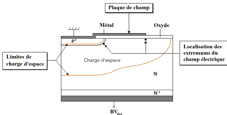
Figure I.16 : Coupe schématique d'une jonction PN équipée d'une plaque de champ [3]
