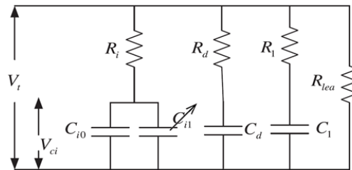
Figure 20. Modélisation d'un supercondensateur par trois branches RC en parallèle. La capacité C_{i1} est proportionnelle à la tension à ses bornes, selon C_{i1} = k.V_{Ci} [60].
