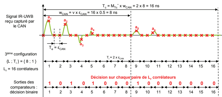
Figure 5.21 – Illustration de la banque de comparateurs après l'étape de corrélation pour estimer le bit reçu sur chaque portion de durée T_i formant la fenêtre temporelle w_{CAN} puis la durée d'un chip T_c .
