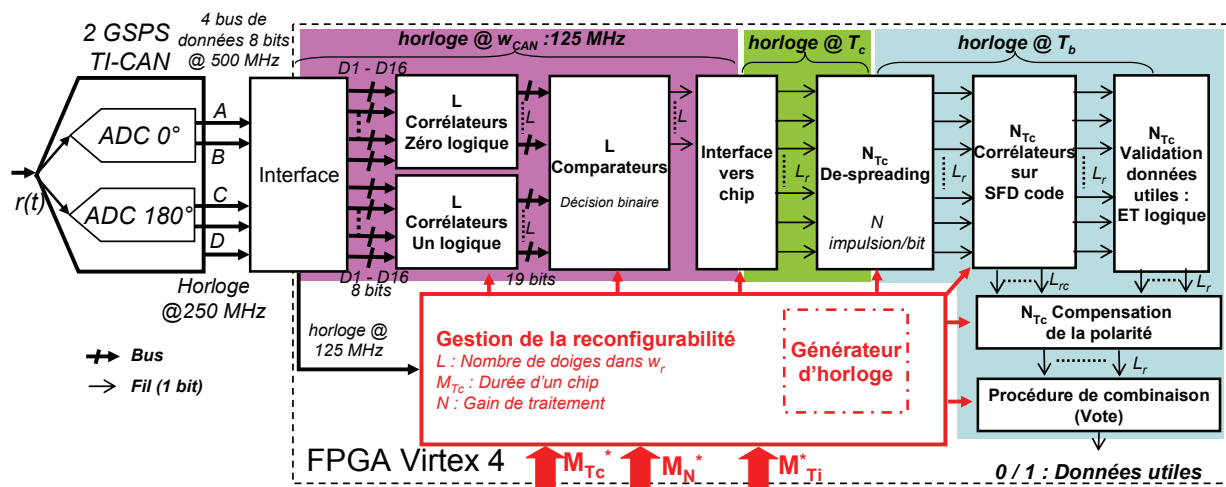
Figure 5.18 – Schéma de principe du circuit numérique de réception Rake IR-UWB BPSK reconfigurable.
