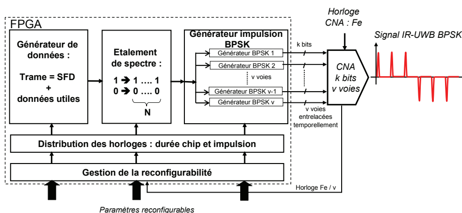
Figure 4.3 – Structure de l'émetteur IR-UWB BPSK reconfigurable proposé construit autour d'un CNA à entrelacement temporel et de cinq fonctions de base.
