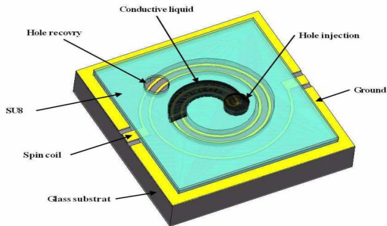
Figure 14 : Représentation du MEMS fluïdique assurant les fonctions d'inductance continument variable.
