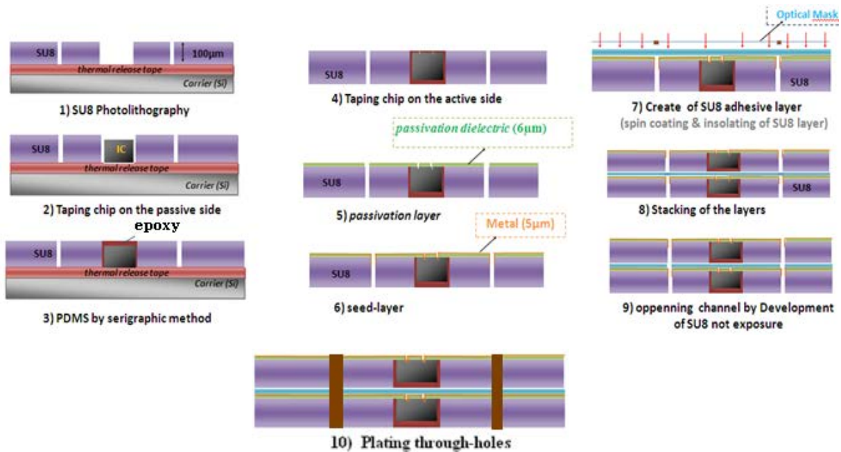
Figure 20 : Description du procédé TPV à base de SU8.
