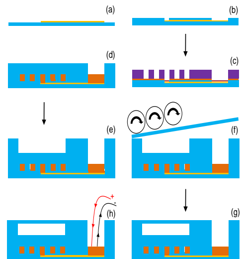
Figure 7. Procédé de réalisation de microsystemes fluidiques comportant des bobines intégrées.
