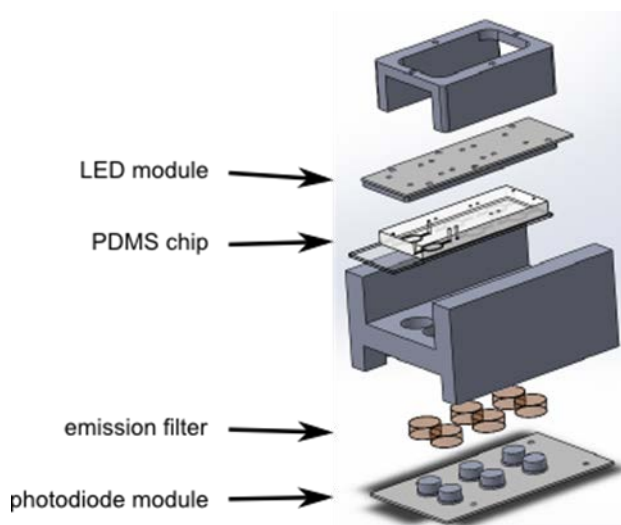
Figure 22 : Représentation de la globalité du système d'évaluation de DBO intégrant la chaîne instrumentale à base de MEMS
