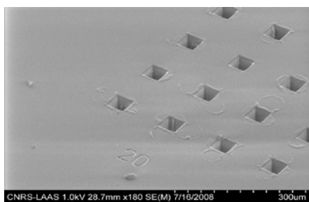
Figure 19 : Photo MEB montrant des trous ( 20\ \mu\text{m} de côté) traversant 500\ \mu\text{m} d'une couche de SU8.
