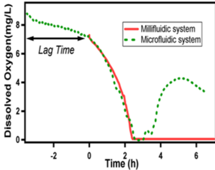
Figure 24 : Courbes représentant la concentration d'oxygène en fonction du temps pour les systèmes microfluidiques et macroscopique
