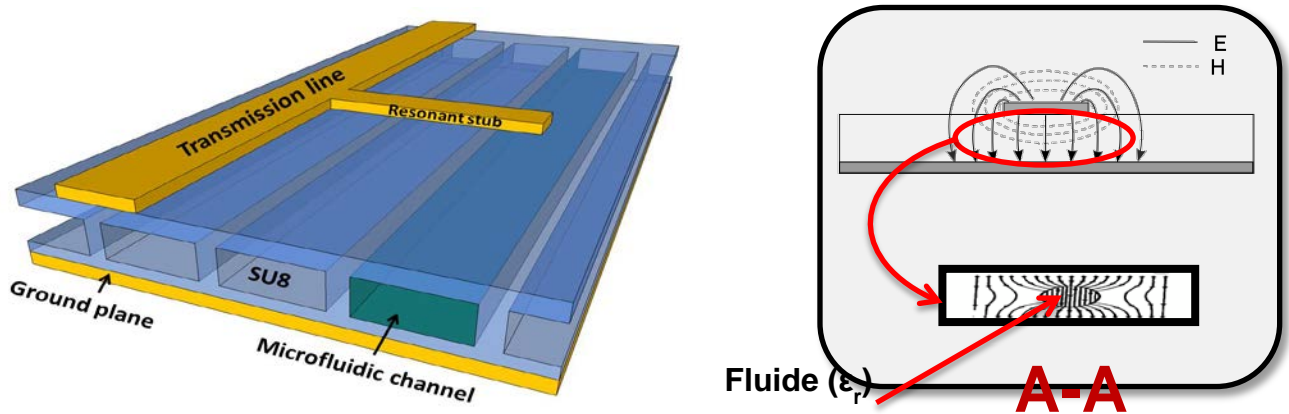
Figure 10 : a) Schéma représentant le dispositif MEMS à réaliser et alliant circuit RF et canaux microfluidiques ; b) interactions fluides/lignes de champs E et H dans les structures tridimensionnelles envisagées.
