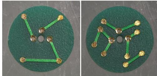
Figure I.21 : Photos du PCB porte-puces : (à gauche) face avant ou côté PyroMEMS ; (à droite) face arrière.
