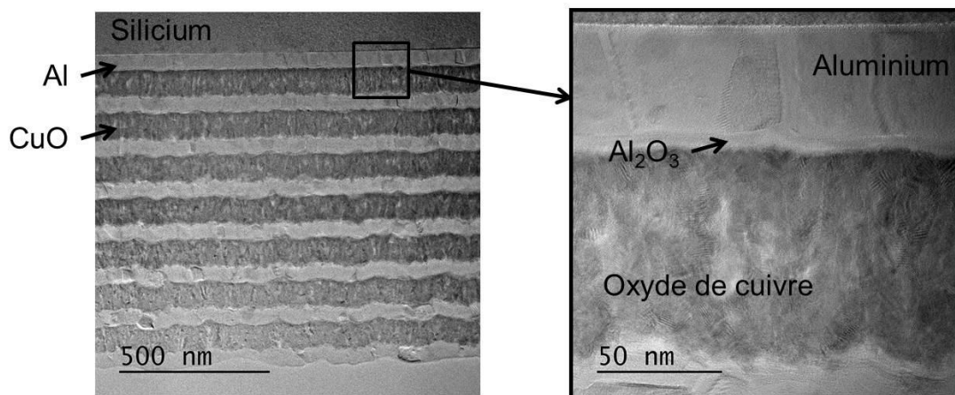
Figure II.25 : (à gauche) Image MET d'un dépôt de 15 couches Al (50 nm) / CuO (100 nm) déposées sur un substrat en silicium ; (à droite) Zoom sur une couche d'Al et de CuO montrant la couche d'oxyde entre l'aluminium et le CuO.
