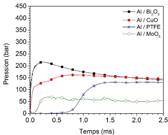
Figure III.15 : Evolution temporelle de la pression an bombe manométrique dans un volume de 9 \text{ mm}^3 pour les différents couple de nanothermite compacté à 30 % TMD.
