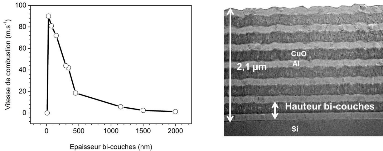
Figure 11.19 : (à gauche) Courbe de la vitesse de combustion en fonction de l'épaisseur d'un bi-couches pour une hauteur de nanothermite de 2,1 \mu\text{m} constante ; (à droite) illustration d'un bi-couches sur un dépôt de 2,1 \mu\text{m} .
