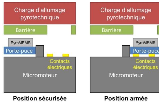
Figure I.17 : Schématisation de l'armement mécanique de l'IFI.
