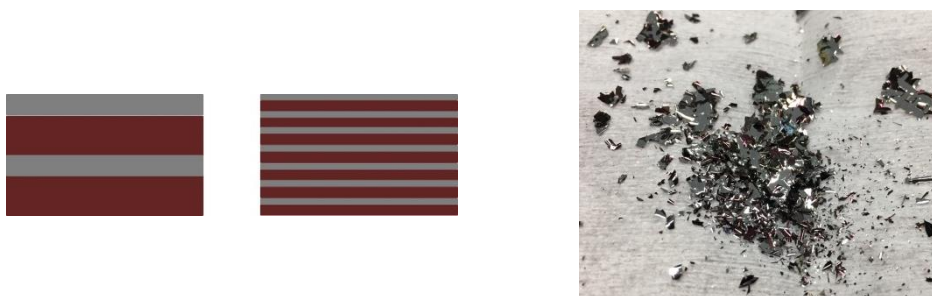
Figure III.2 : Schéma démonstratif de la différence entre des couches micrométriques (à gauche) et nanométriques (au centre) ; (à droite) Photo de flocons Al / CuO.
