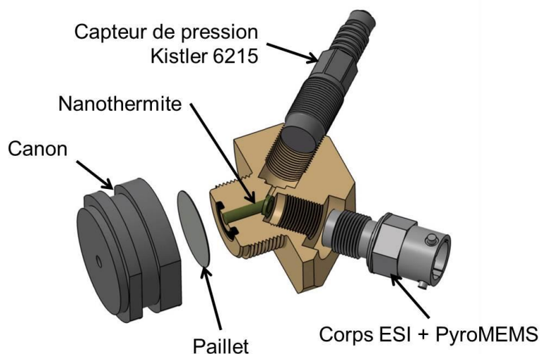
Figure III.23 : Vue éclatée en 3D du canon, du paillet et de la chambre de combustion (en coupe) intégrant de la nanohermite, un initiateur et un capteur de pression Kistler 6215.
