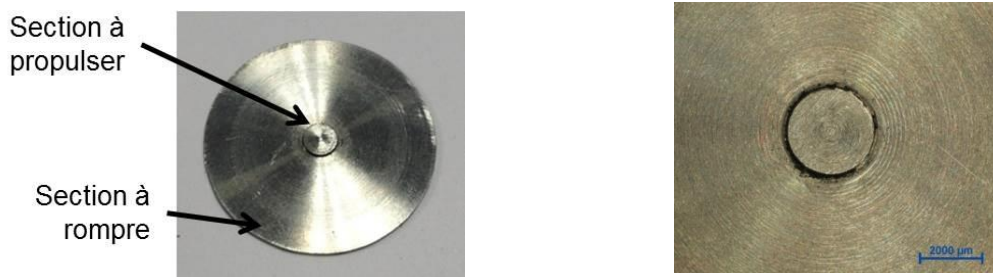
Figure IV.5 : (à gauche) Photo vue d'ensemble du paillet ; (à droite) Zoom montrant la partie propulsée [IV.1].
