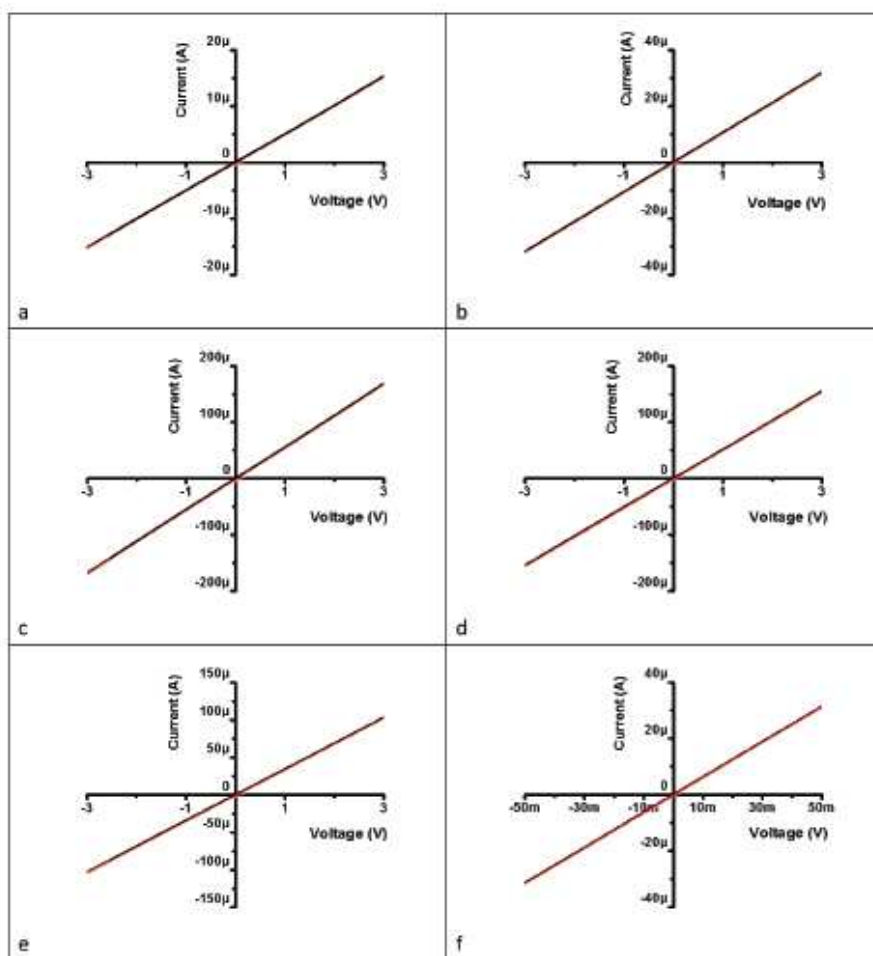
Caractéristiques électriques I(V) à température ambiante de six capteurs différents intégrant ds NTCs oxydés. Les résistances varient entre 2 et 200 \text{k}\Omega .
