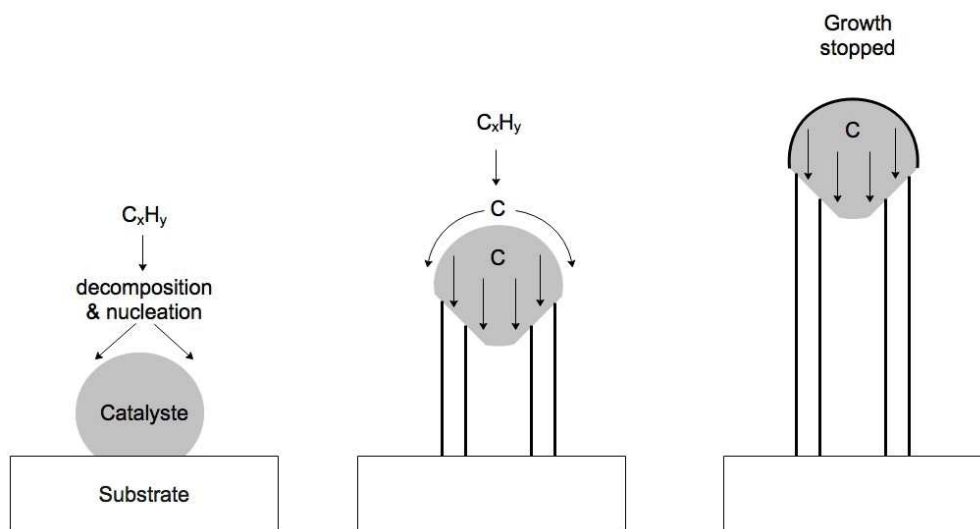
Croissance des nanotubes de carbone sur particule métallique : (a) «tip-growth model», (b) «base-growth model»
