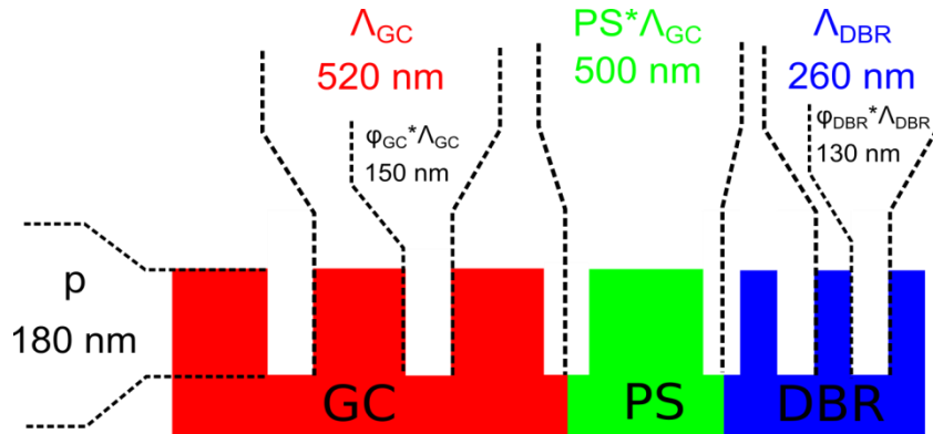
Figure 38 : Schéma récapitulatif des valeurs typiques des caractéristiques des trois constituants du CRIGFs : le réseau central (GC), la zone d'adaptation de phase (PS) et le réflecteur de Bragg (DBR).
