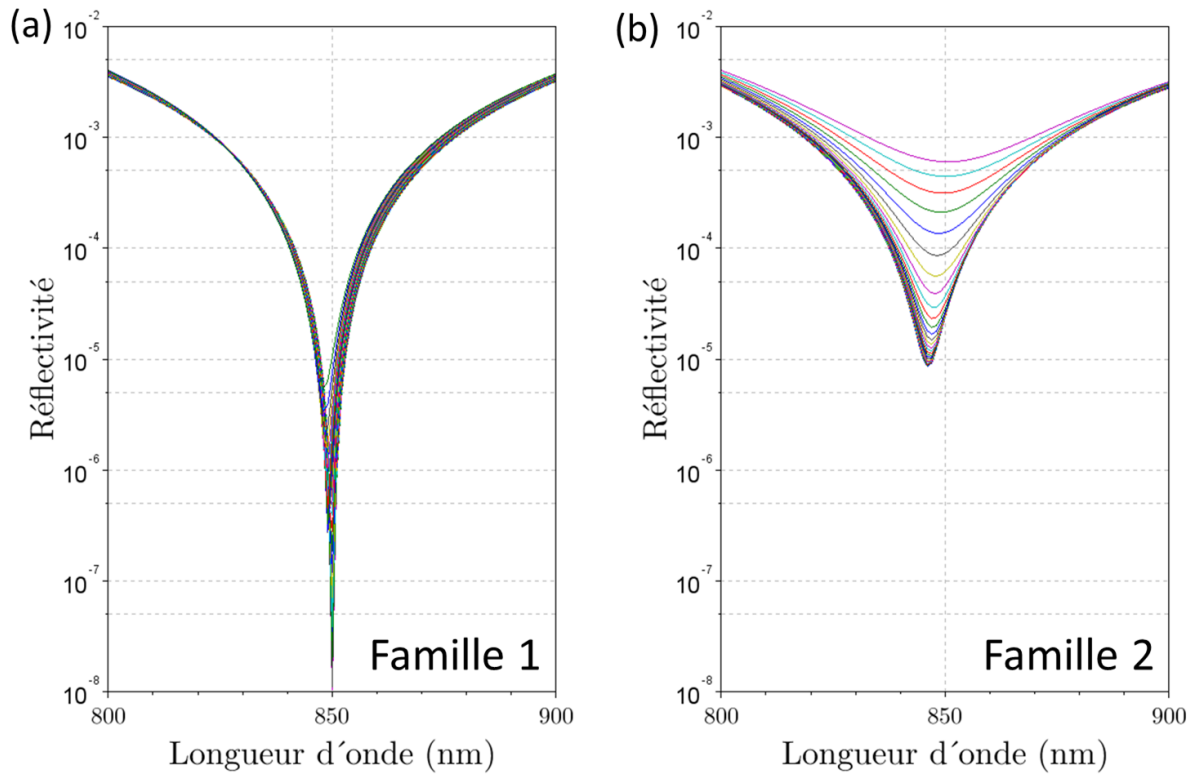
Figure 106 : Spectres de réflectivité des empilements moyens (a) de la famille 1 et (b) de la famille 2.
