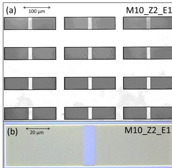
Figure 82 : (a et b) Image de CRIGFs structurés dans la résine NILUV avec un moule souple dupliqué à partir du moule dur M10 ( e_{M10} = 83 nm).
