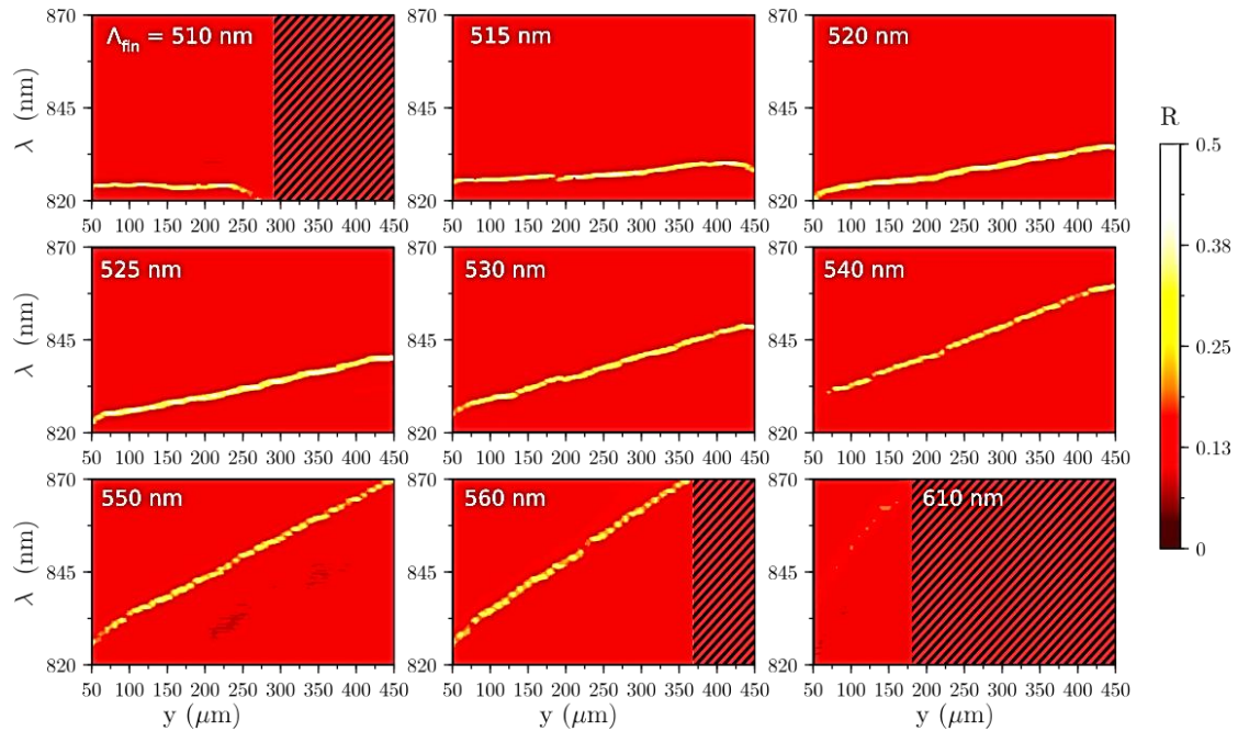
Figure 134 : Cartographies des spectres de résonance des différents GCRIGFs le long de l'axe y . Les parties hachurées correspondent aux parties défectueuses du composant ou aux réponses spectrales hors gamme de la source laser.
