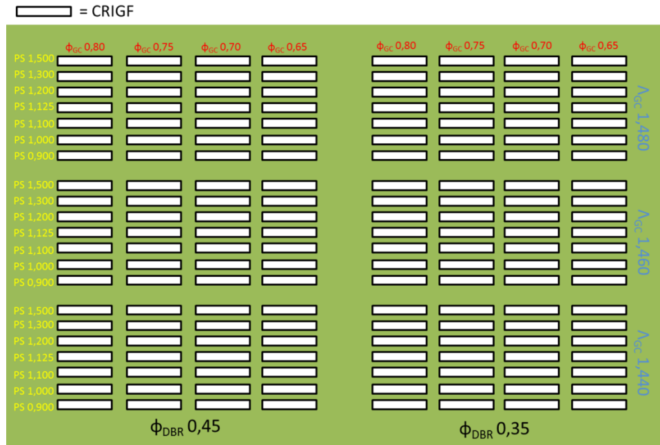
Figure 143 : Schéma représentant un « bloc » de 168 CRIGFs (≈3,6x5,5 mm 2 ). Les différentes caractéristiques géométriques mises en jeu sont : la période du GC ( \Lambda_{GC} ), la zone d'adaptation de phase (PS), le taux de remplissage du GC ( \phi_{GC} ) et le taux de remplissage des DBRs ( \phi_{DBR} ).
