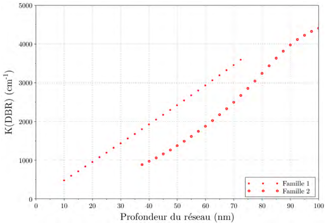
Figure 107 : Coefficient de couplage dans les zones DBR ( K_{DBR} ) pour les deux familles de solution en fonction de l'épaisseur de la couche réseau.
