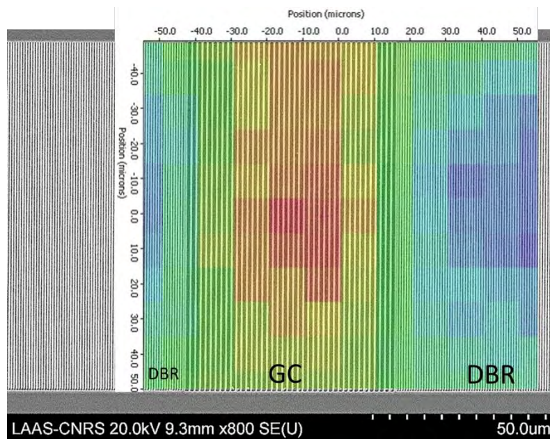
Figure 162 : Cartographie de la réflectivité maximale en fonction du positionnement sur une image MEB du CRIGF MIR.
