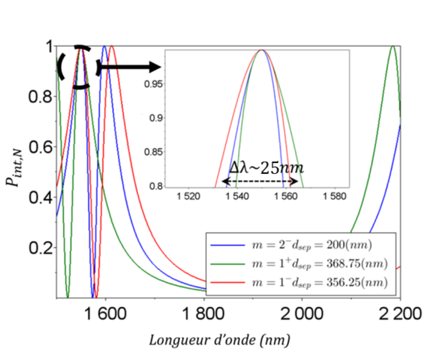
Fig. 5.8. Evolution de la puissance intra-cavité normalisée P_{int,N} en fonction de la longueur d'onde pour différents ordres de couplage critique ( 1^- , 1^+ et 2^- ) et leur épaisseur de séparation, correspondant à une même longueur de couplage L_{min} \sim 22 \mu\text{m} .
