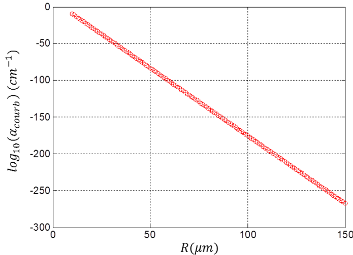
Fig. 3.21 : Evolution des pertes par courbure du mode \text{TE}_0 des parties courbées des résonateurs rectangulaires arrondis aux angles avec h=0,5 \mu\text{m} et w=1,25 \mu\text{m} en fonction du rayon externe R . Calcul réalisé à partir de l'équation (3.7) [27], [22].
