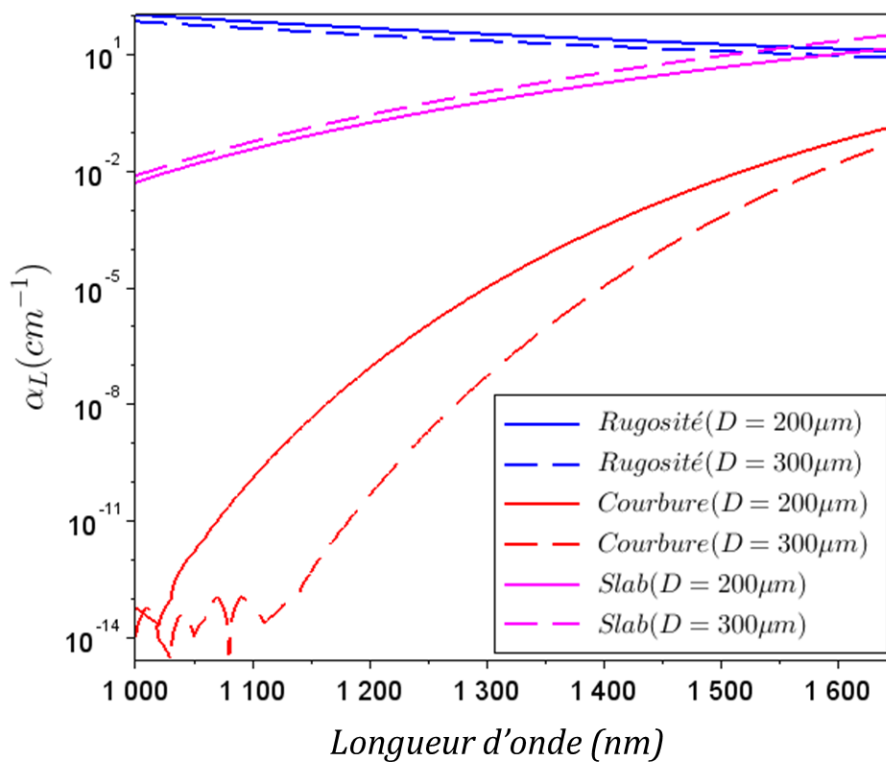
Fig. 3.29 : Evolution en longueur d'onde des différentes contributions aux pertes internes d'un disque AlGaAs/AIOx de 200 \mu\text{m} de diamètre (courbes en trait plein) et de 300 \mu\text{m} de diamètre (courbes en pointillés) correspondant aux indices effectifs représentés sur la figure 2.19.
