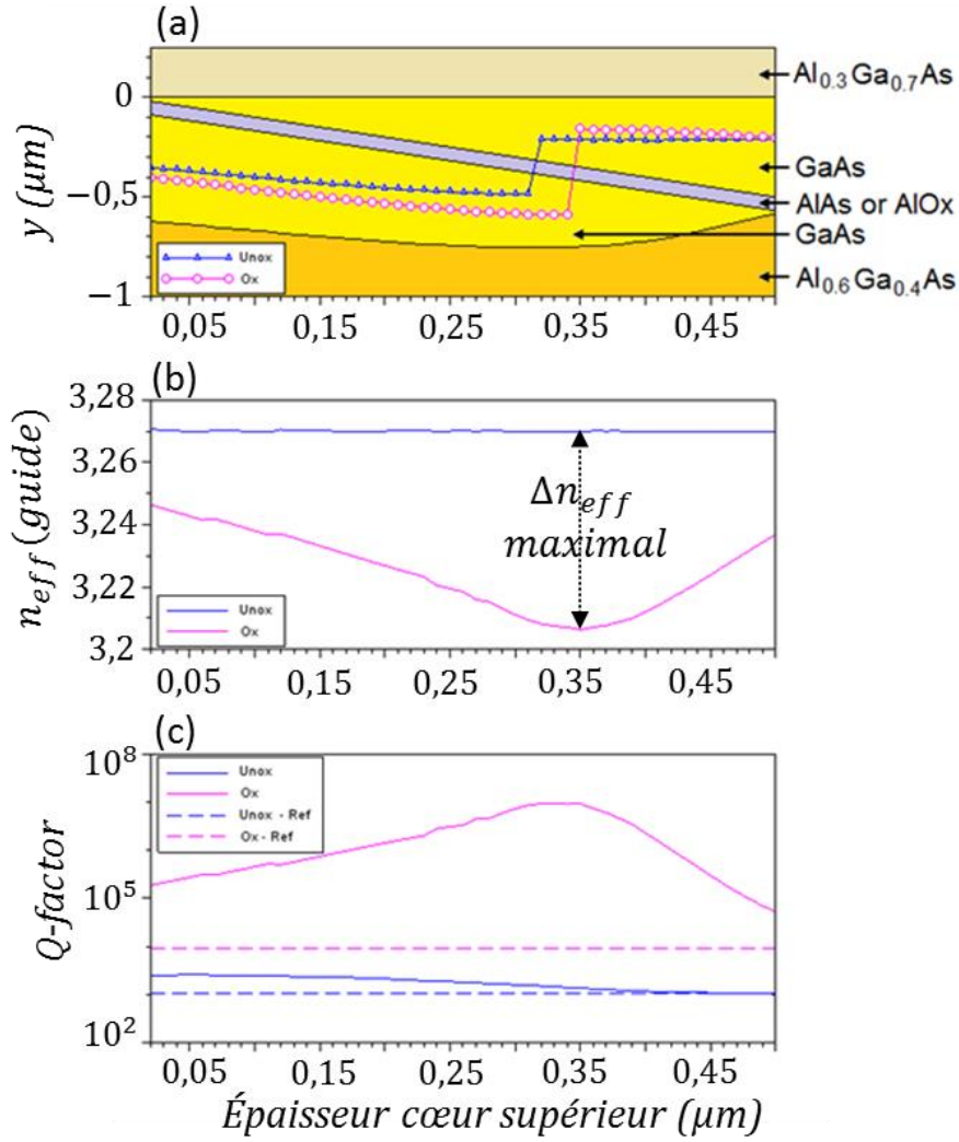
Fig. 5.30: Conception du guide d'accès double cœur pour résonateurs de seconde génération de 300 \mu\text{m} de diamètre. (a) Position verticale de la couche centrale d'oxyde (bande grise) et du maximum du profil de mode (cas oxydé : ligne et cercles magenta, cas non-oxydé : ligne et triangles bleus) (b) Indice effectif du mode fondamental vertical correspondant aux configurations présentées au-dessus (cas non-oxydé en bleu et oxydé en magenta) (c) facteurs de qualité correspondants, en fonction de l'épaisseur du cœur supérieur.
