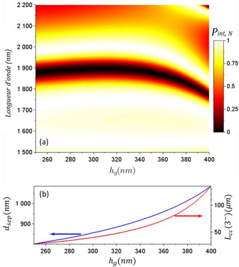
Fig. 5.20. (a) Evolution du spectre de puissance intra-cavit e normalis ee, en fonction de l' paisseur du guide d'acc es h_g (entraignant une variation de \delta^2 ) dans le cas o  F est achromatique. (b) : Evolution de la distance de s paration   laquelle se produit le sc nario o  F est achromatique (courbe bleue) et de la longueur de couplage critique correspondante (courbe rouge) en fonction de l' paisseur du guide d'acc es h_g .
