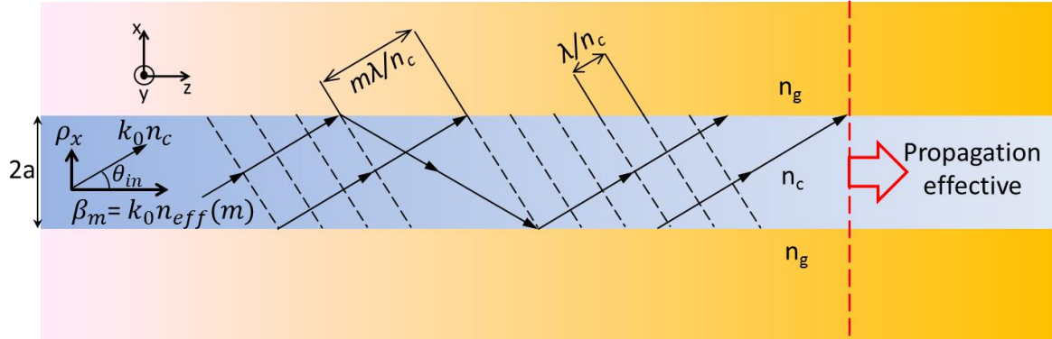
Fig 2.1 Schéma des réflexions totales internes des rayons lumineux et des fronts d'ondes perpendiculaires correspondants dans un guide d'onde. Un mode propre ne s'établit dans la structure que si un nombre entier m de longueurs d'ondes sépare deux séries de fronts d'ondes parallèles après chaque réflexion, permettant à ces derniers d'interférer constructivement. La propagation des rayons en « zig-zag », due aux multiples réflexions aux interfaces, s'effectue globalement selon l'axe z . C'est la signification de la constante de propagation effective \beta_m .
