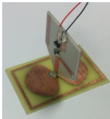
Figure II-51. Rectenna réalisée
