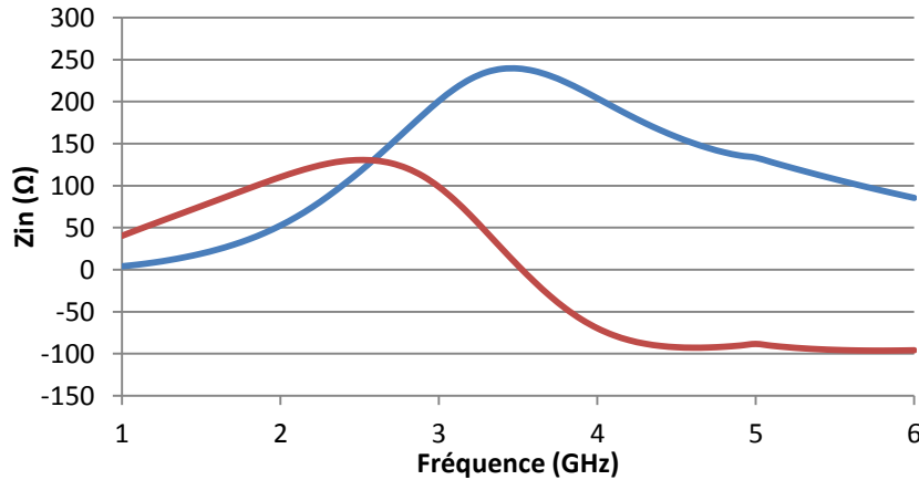
Figure III-25. Impédance d'entrée co-simulée ( R = 500\Omega et PR_{Fin} = 0\text{ dBm} )
