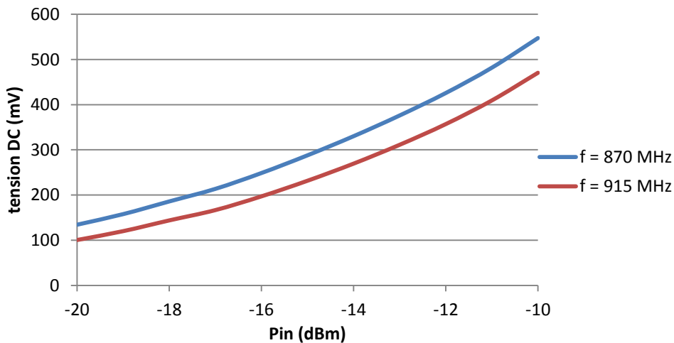
Figure IV-4. Tension DC récupérée en fonction de la puissance RF, R = 10 k \Omega
