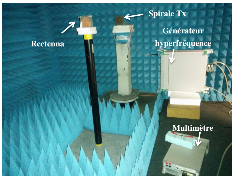
Figure III-31. Banc de mesure pour la rectenna large bande
