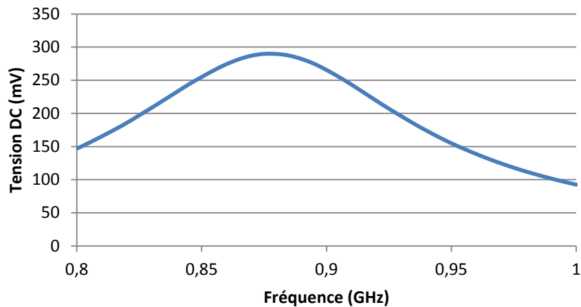
Figure IV-3. Tension DC récupérée en fonction de la fréquence, R = 10 k \Omega et Pin = -15 dBm
