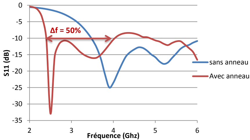
Figure II-45. Coefficient de réflexion pour l'antenne DA sans anneau (bleu) et avec anneau (rouge)
