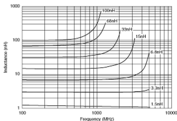
Figure I-33. Caractéristique d'inductances Murata en fonction de la fréquence [38]
