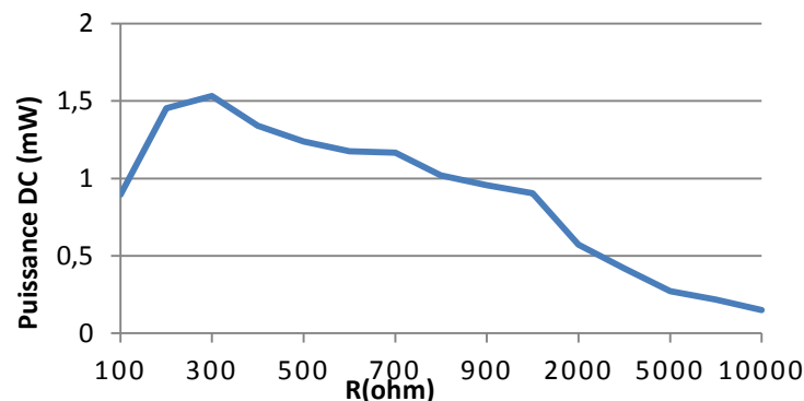
Figure III-12. Puissance DC en fonction de la charge pour f = 12 GHz et E = 48 V/m
