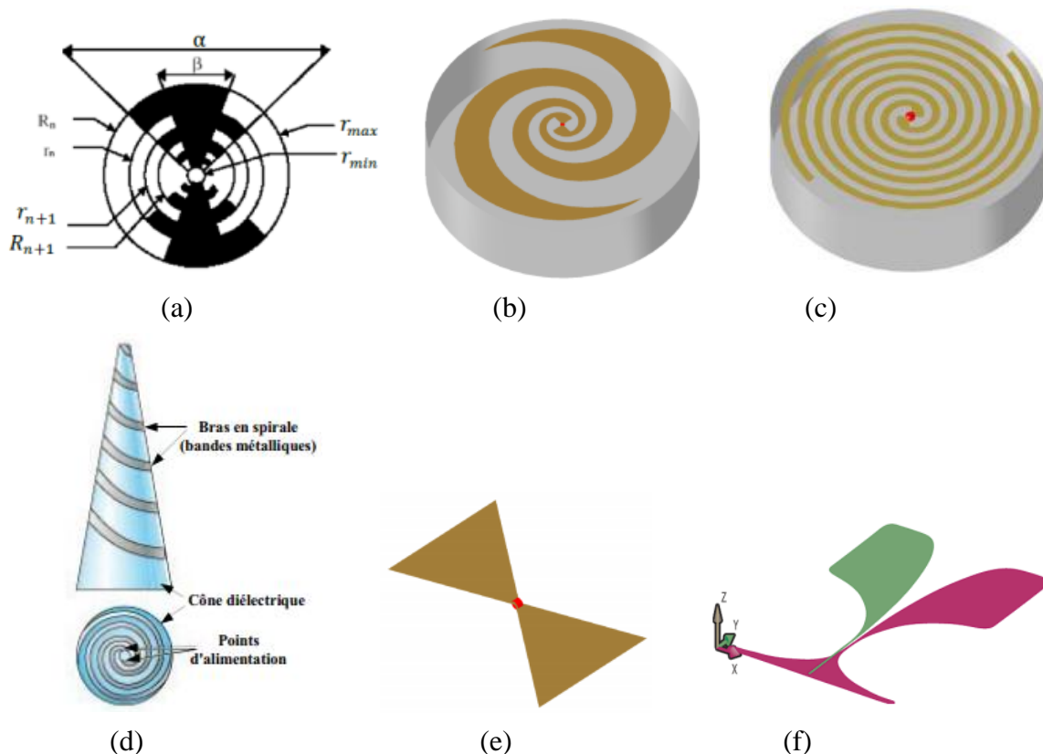
Figure III-14. (a) Antenne Log-périodique trapézoïdale (b) Antenne Log-spirale (c) Antenne Spirale d'Archimède (d) Antenne conique (e) antenne bow-tie (f) Antenne Vivaldi antipodale
