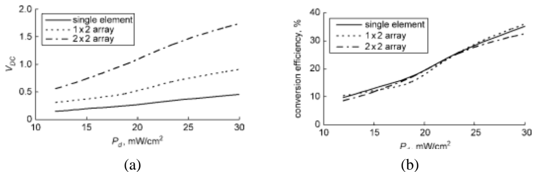
Figure I-55. Résultats de la rectenna [54] (a) tension DC (b) efficacité
