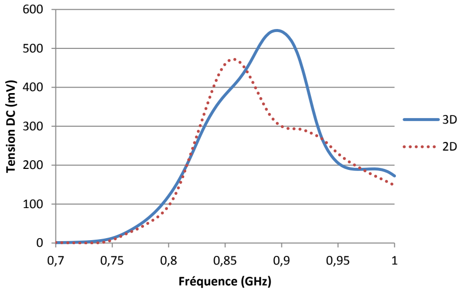
Figure IV- 14. Tension DC en fonction de la fréquence pour une charge de 10 k \Omega
