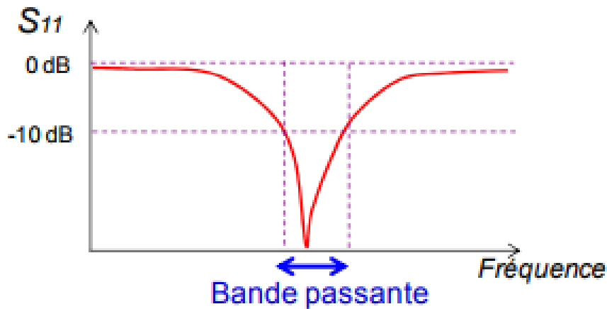
Figure I-27. Coefficient de réflexion en fonction de la fréquence, seuil de BP défini à -10dB [31]
