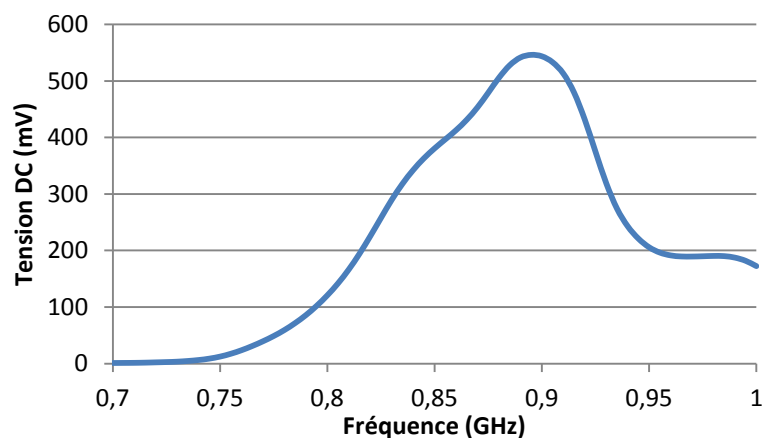
Figure IV-11. Tension DC récupérée à 900 MHz pour une charge de 10 \text{ k}\Omega en fonction de la fréquence
