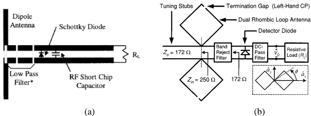
Figure I-30. Rectenna à polarisation (a) linéaire [33] (b) circulaire [35]
