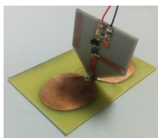
Figure II-40. Rectenna réalisée
