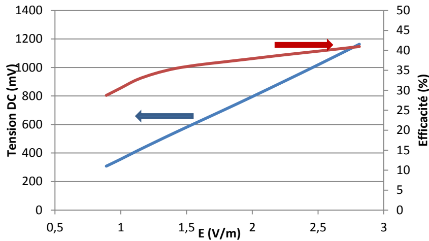
Figure IV-12. Tension DC et efficacité de conversion en fonction du champ électrique incident
