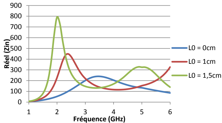
Figure III-27. Partie réelle de l'impédance en fonction de la fréquence pour différentes valeurs de L_0 ( R = 500 \Omega et PR_{Fin} = 0 \text{ dBm} )
