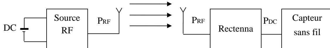
Figure I-13. Architecture d'un système de TESH
