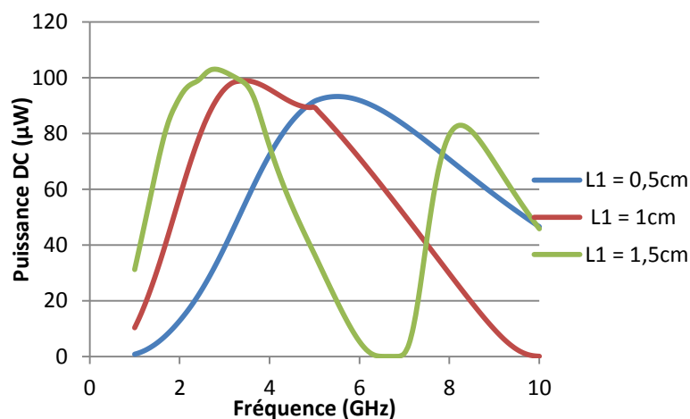
Figure III-28. Puissance DC simulée en fonction de la longueur L_1 ( R = 500 \Omega et PR_{Fin} = 0 \text{ dBm} )
