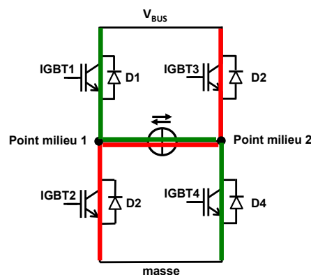
Figure 72 : commande diagonale des bras de pont (conditions de fonctionnement statique)
