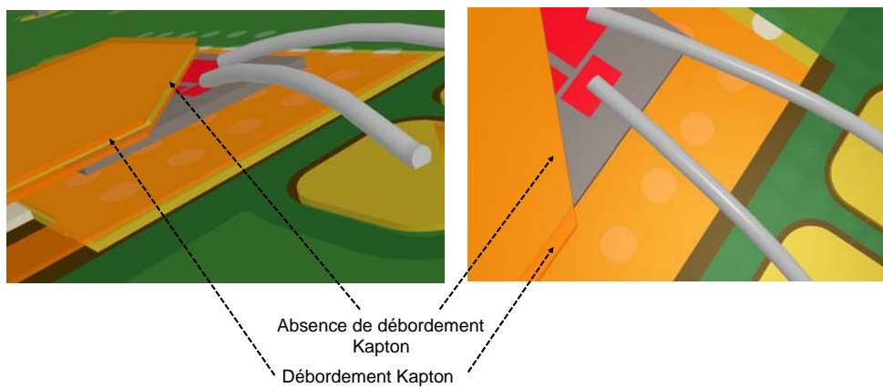
Figure 166 : zoom sur la région de connexion filaire grille et source kelvin de la puce high-side
