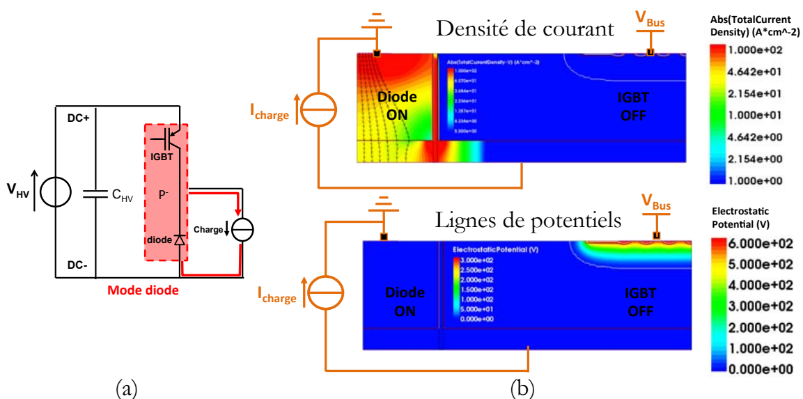
Figure 125 : (a) mode Diode de la cellule buck , (b) observation des densités de courant et des lignes équipotentiels pour le mode Diode
