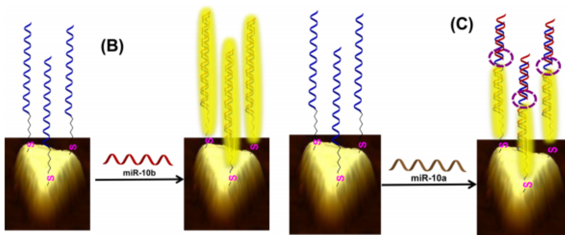
Figure 1-26 : détection de séquences miARNs par SPR via l'utilisation de nanoprismes en or sur lesquels sont greffées des sondes thiolées complémentaires à une séquence miARN spécifique (miR-10b). Les auteurs montrent ici l'effet de la présence d'un nucléotide non apparié avec la séquence cible miR-10a détection. 52
