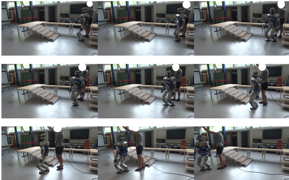
FIGURE 7.4 – Captures du mouvement corps complet exécuté sur le robot HRP-2 pour le scénario de navigation sur sol plat.
