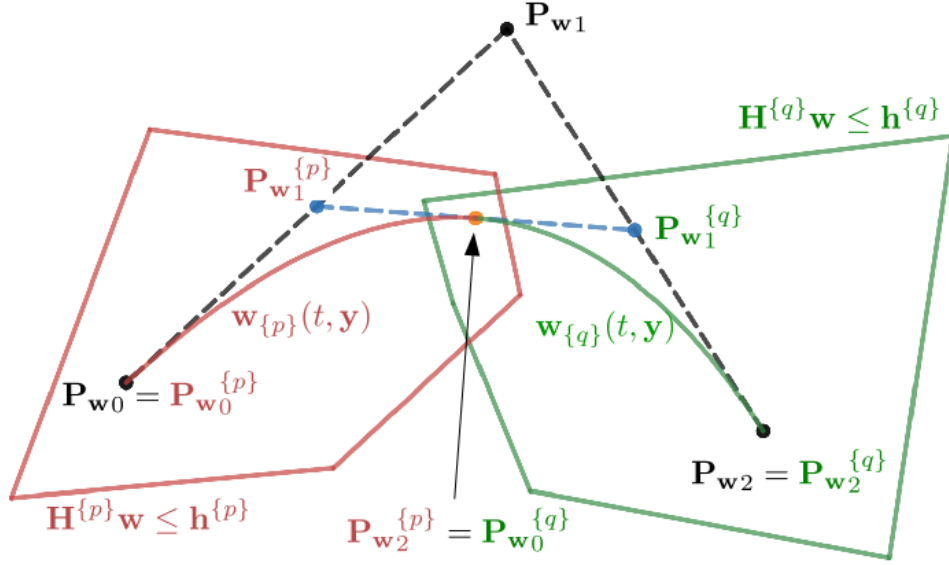
FIGURE 5.4 – Exemple de décomposition de la courbe \mathbf{w} de degré 2 définie par les points de contrôle \mathbf{P}_{w_i} (en noir), à l'instant de transition t = T^{\{p\}} (point orange). La courbe est décomposée en deux courbes de degré 2 également, \mathbf{w}_{\{p\}} définie par les points de contrôle \mathbf{P}_{w_i}^{\{p\}} (en rouge) et \mathbf{w}_{\{q\}} définie par les points de contrôle \mathbf{P}_{w_i}^{\{q\}} (en vert). Chacun de ces ensembles de points de contrôle est alors contraint à satisfaire les contraintes de la phase de contact correspondante. Le résultat est que la courbe satisfait les contraintes correspondantes à la phase de contact courante à chaque instant. On peut noter que les points de contrôle de la courbe originale ne sont pas contraints à satisfaire les contraintes.
