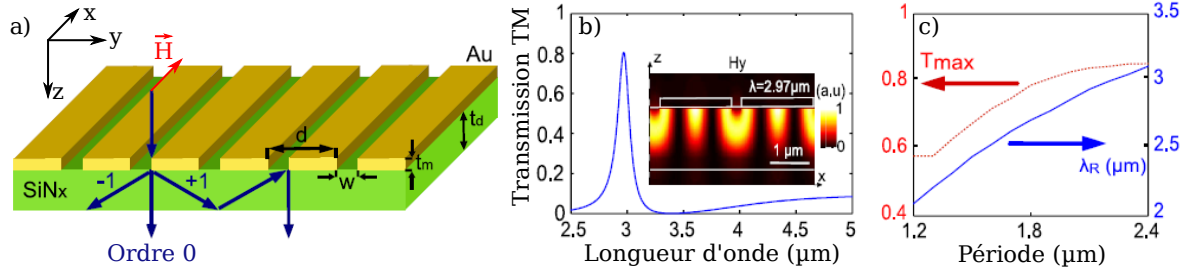
FIGURE 1.15 – Tiré de [78]. a) Structure du réseau suspendu. Les paramètres sont : d = 2110 nm, w = 215 nm, t_m = 70 nm, t_d = 540 nm. b) Spectre en transmission du réseau pour une incidence TM, avec représentation de l'amplitude du champ |H_y|^2 dans le réseau à la résonance ( \lambda_r = 2.97 \mu\text{m} ). c) Illustration de l'accordabilité du filtre avec la période.
