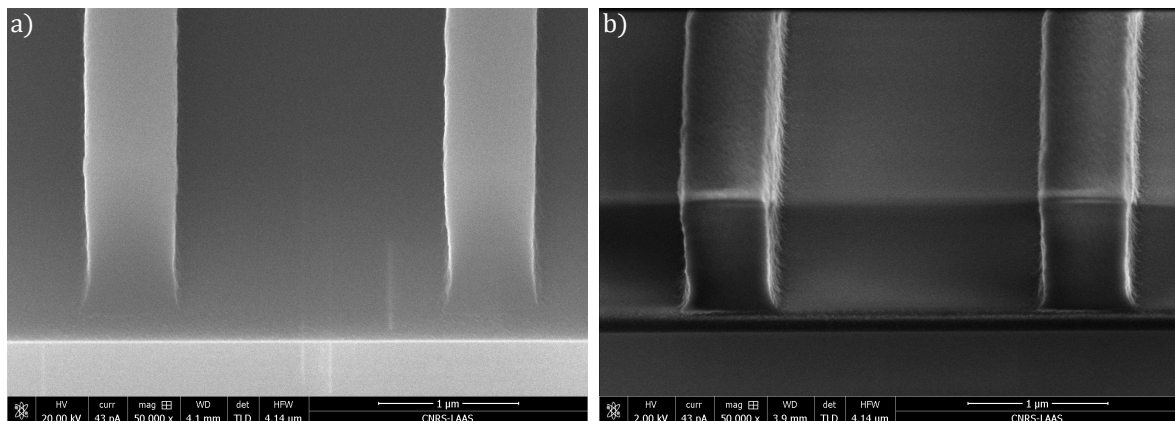
FIGURE C.3 – Vue MEB en coupe de motifs insolés sur wafer 6 pouces dans les mêmes conditions d'exposition (Dose égale à 1100 \text{ J}/\text{m}^2 et focus de -0,2 \mu\text{m} ), mais pour différents réglages du MEB (a) V_{\text{acc}} = 20 \text{ kV} , I = 86 \text{ pA} , et b) V_{\text{acc}} = 2 \text{ kV} , I = 43 \text{ pA}
