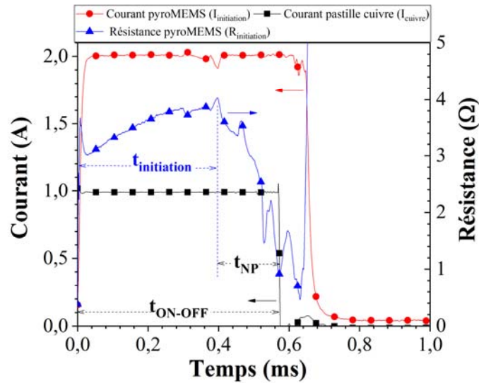
Figure IV.25 : Evolution du courant dans le pyroMEMS et aux bornes de la piste en cuivre, pendant le test de fonctionnement du sectionneur.
