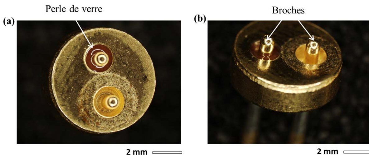
Figure III.2 : (a) Vue de dessus et de (b) côté de la traversée de verre.
