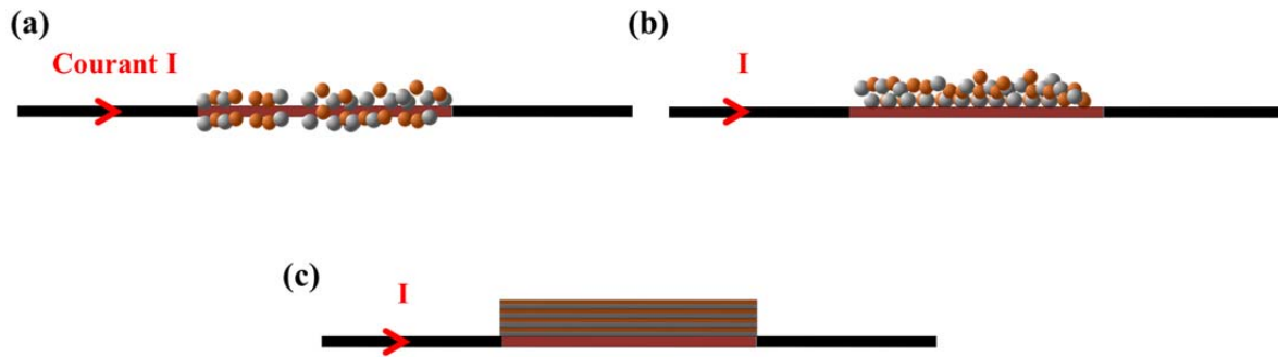
Figure I.12 : Schéma de l'initiation électrique. (a) Fil avec une couche de nanothermites. (b) Fil avec une composition en poudres au-dessus et (c) fil avec une thermite multicouches.
