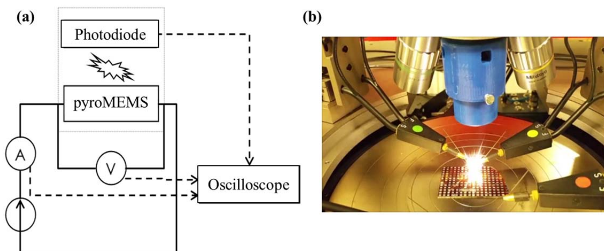
Figure II.10 : Schéma du montage électrique (a) utilisé pour caractériser les initiateurs et (b) photo pendant une mesure.
