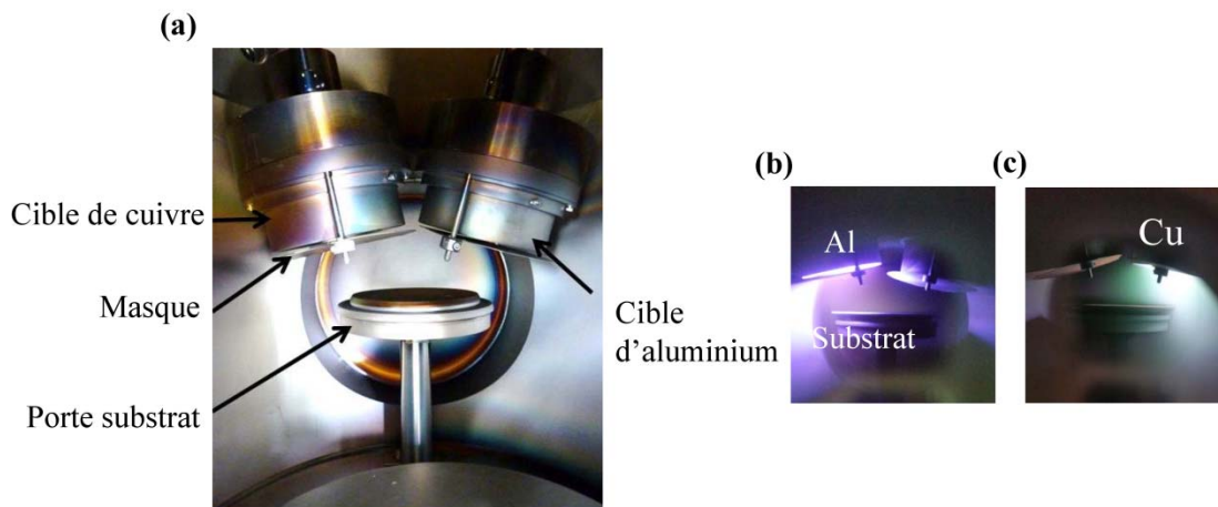
Figure I.5 : (a) Photo de l'intérieur de la chambre de dépôt montrant la configuration. Photos de l'intérieur de la chambre de dépôt pendant un plasma d'Ar (b) et un plasma Ar + O 2 (c).
