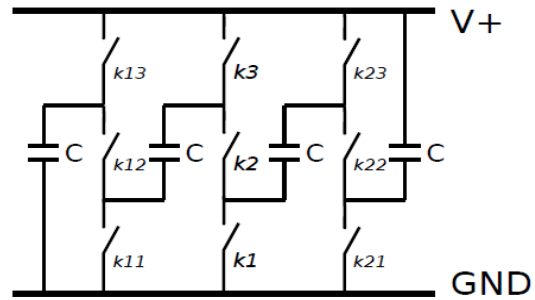
Figure 1-25 : Topologie alternative pour le stockage de l'énergie.
