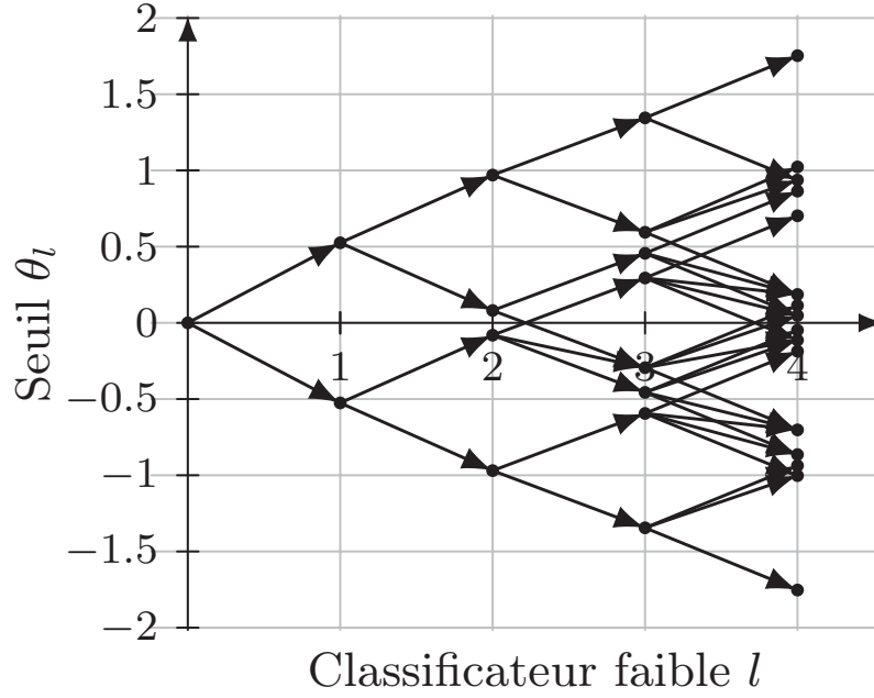
FIGURE 2.8 – Le graphe de seuil de la Figure 2.6 après appliquer les Propositions 2.2 et 2.3.
