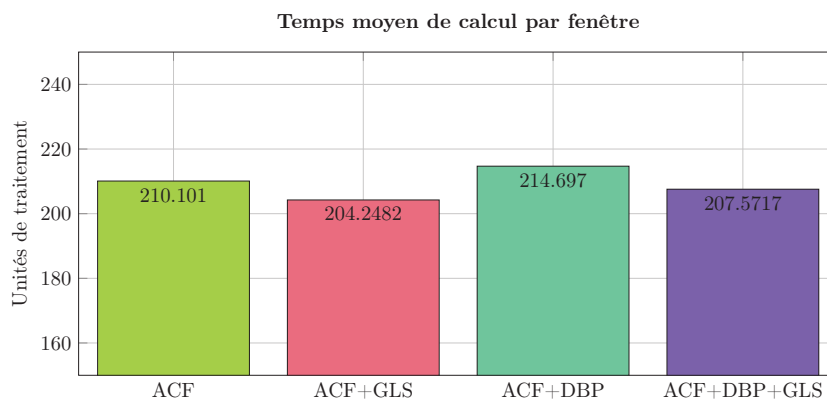
FIGURE 2.14 – Valeurs de la fonction objectif c'est-à-dire temps moyens de calcul des évaluations par fenêtre sur la base INRIA.
